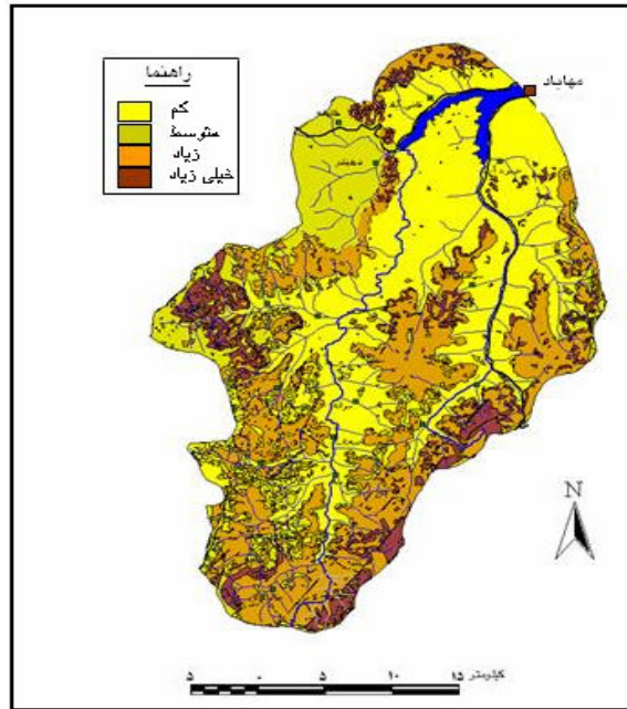
شکل ۴- نقشه حساسیت نواحی مختلف حوضه آبریز رود مهاباد به تولید رسوب
