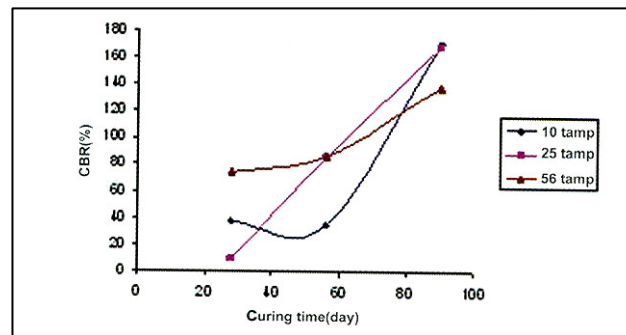
نمودار ۱۱- تغییرات CBR و زمان عمل آوری در کوبشهای متفاوت برای نمونه محتوی ۶٪ آهک زنده
