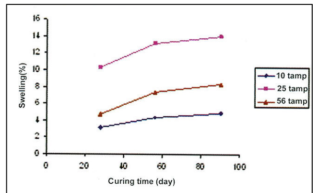
نمودار ۷- تغییرات میزان تورم نمونه‌ها و زمان عمل آوری در تعداد ضربات کوبش متفاوت و نمونه محتوی ۶٪ آهک زنده
