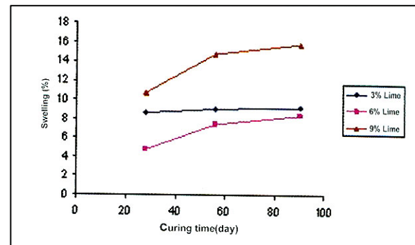
نمودار ۹- تغییرات میزان تورم و زمان عمل آوری در نمونه محتوی درصدهای مختلف آهک زنده و ۵۶ ضربه کوبش
