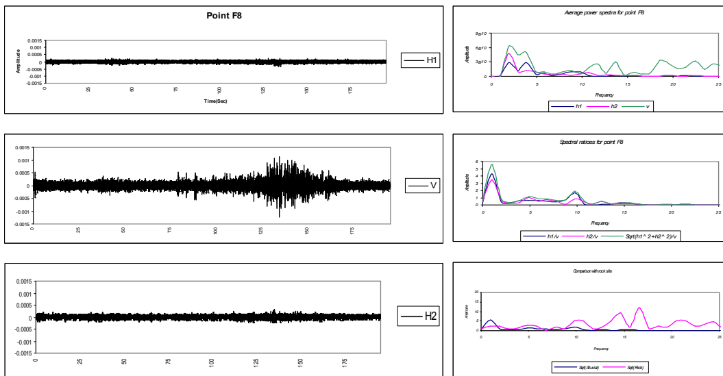
شکل ۳ - سریهای زمانی مربوط به نقطه F_8 و طیف حاصل از پردازش آن
