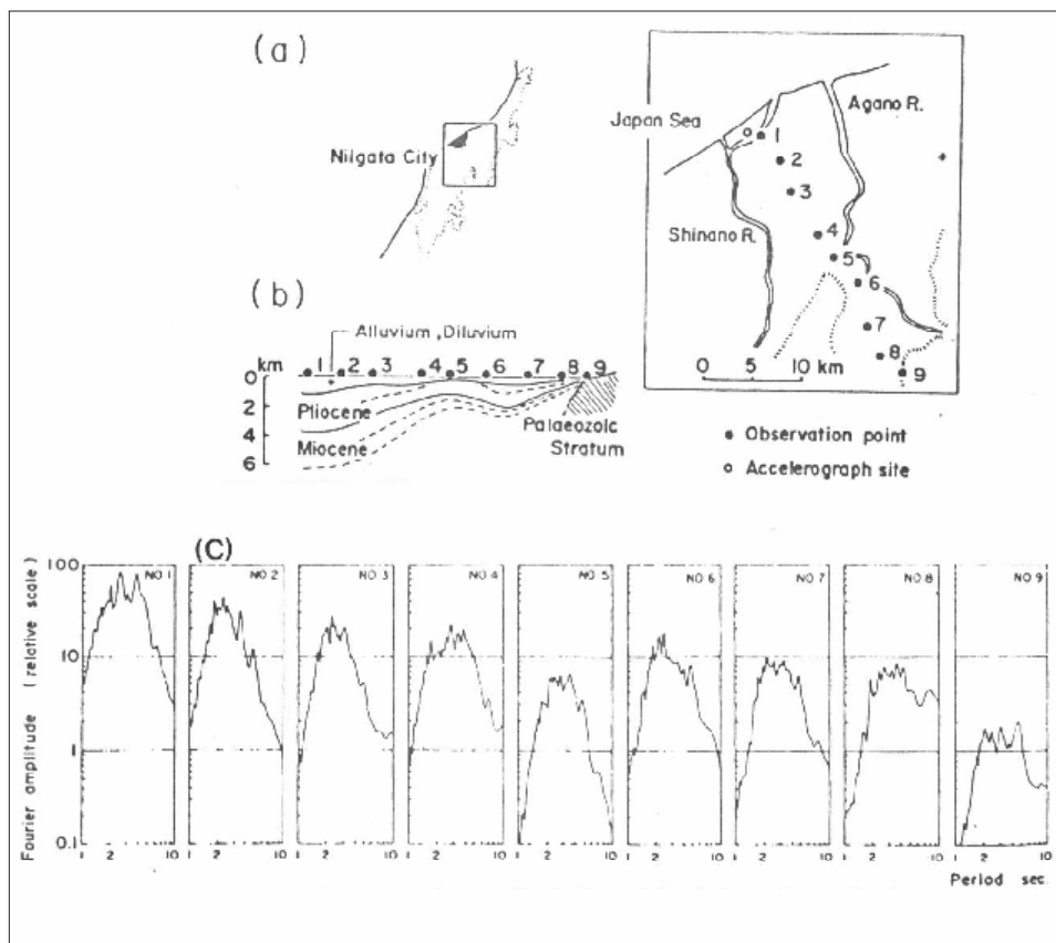
شکل ۱- (a) موقعیت نقاط اندازه‌گیری مایکروترمورها در دشت Niigata (b) شرایط زیر سطحی در طول نیمرخ (c) نمایش متوالی از طیفها در طول نیمرخ (Kagami et al., 1996)
