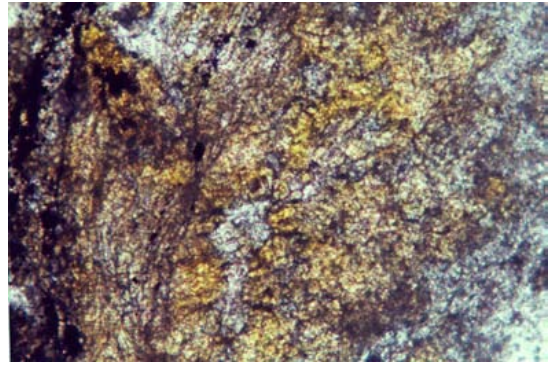
شکل ۱۲- مقطع میکروسکوپی از یک نمونه متاآندزیت بازالتی پیرامون گرانیت که در اثر عملکرد سیالها، کانیه‌های کدر آن شسته شده و در بخشهای دارای کرنات به صورت مگنتیت نهشته شده است.
