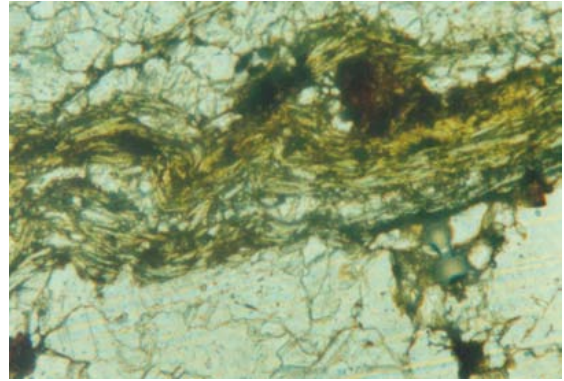
شکل ۶- مقطع میکروسکوپی از شکل ۵ در نور PPL با بزرگنمایی ۲۰ در نور عبوری. لامینه آتشفشانی بیشتر به کلریت تبدیل شده و کانه‌ها همراه با برگراگی کلریت و به تبع از آن چین خورده‌اند.
