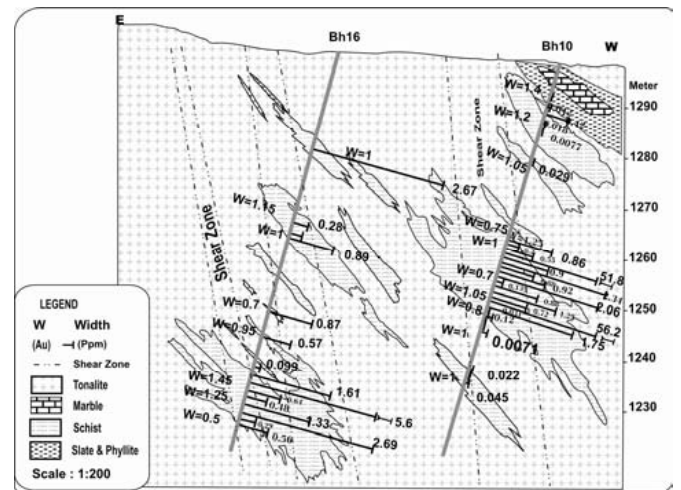
شکل ۳- نمایش تغییرات مقدار طلا در نیمخ چاههای Bh16-Bh-10 (ترابیان، ۱۳۸۳).
