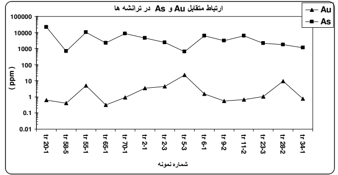
شکل ۵- رابطه متقابل Au و As و همبستگی نسبی و مثبت بین این دو عنصر (ترابیان، ۱۳۸۳).
