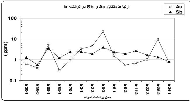
شکل ۶- ارتباط متقابل عناصر Au و Sb در ۱۴ ترانشه سطحی (ترابیان، ۱۳۸۳).
