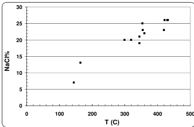
شکل ۸- نمودار دمای همگن شدن و میزان املاح میانبارهای سیال طر قبه کانی سازی طلای طر قبه (ترابیان، ۱۳۸۳).
