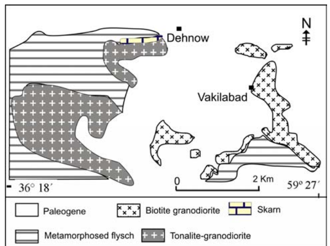
شکل ۹- نقشه رخنمون توده های نفوذی در محدوده وکیل آباد - طر قبه - دهنو.
