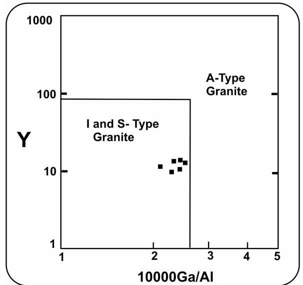
شکل ۱۱- نمودار نسبت 10000Ga/Al در برابر Y (کریم پور و دیگران، ۱۳۸۴).
