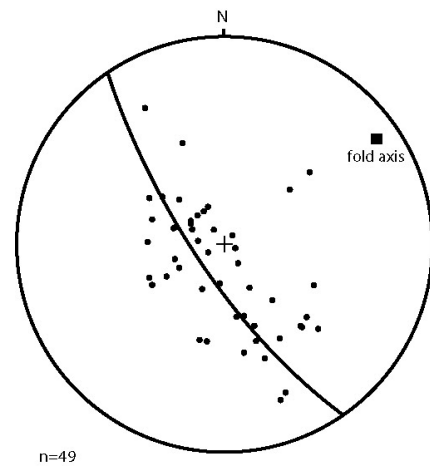
شکل ۶) تصویر استریوگرافیک قطب لایه‌های چین خورده بر اثر F3
