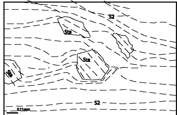
شکل ۳) تصویر نمادین رسم شده از روی تصویر میکروسکوپی که در آن برگوارگی چیره سنگ (S2) پرفیروبلست‌های استارولیت با انحراف از روند فعلی آنها دنبال می‌شود. این امر نشانگر تبلور این کانی‌ها به صورت همزمان با S2 است.
