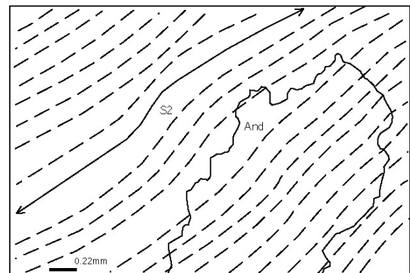
شکل ۴) تصویر نمادین رسم شده از روی تصویر میکروسکوپی که در آن کانی آندالوزیت دارای آثار درونباری همخوان با برگوارگی احاطه کننده آن (S2) است. این امر نشانگر تشکیل آن پس از تشکیل برگوارگی چیره سنگ (S2) است.
