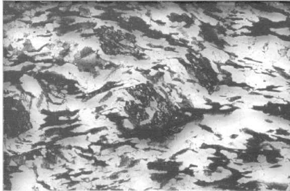
شکل ۳) تصویر نمادین رسم شده از روی تصویر میکروسکوپی که در آن برگوارگی چیره سنگ (S2) پرفیروبلست‌های استارولیت با انحراف از روند فعلی آنها دنبال می‌شود. این امر نشانگر تبلور این کانی‌ها به صورت همزمان با S2 است.
