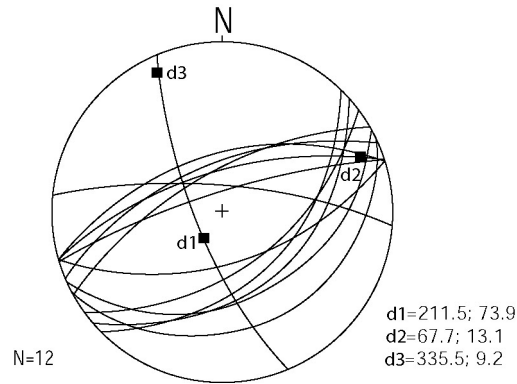
شکل ۸) تصویر استریوگرافیک گسل‌های مزدوج عادی ایجاد شده در اثر رویداد دگر شکلی D4.
