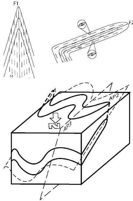
شکل ۵) سیر تحول ساختاری نمادین منطقه مورد بررسی الف) ایجاد یک تاقدیس ایستاده در اثر رویداد دگرشکلی (F1) D1. ب) ایجاد یک چین یال موازی برگشته در اثر رویداد دگر شکلی (F2) D2. ج) نمودار بلوکی نمادین ساختمان‌های بزرگ مقیاس منطقه مورد بررسی.
