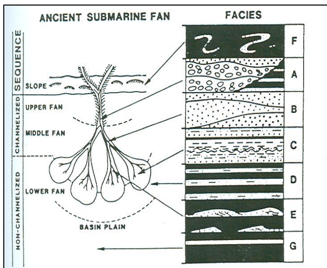
شکل ۱۱ - تقسیم بندی یک بادزن زیر دریایی و رخساره های همراه با هر بخش (نقل از Moiola & Shanmugam, 1988).
