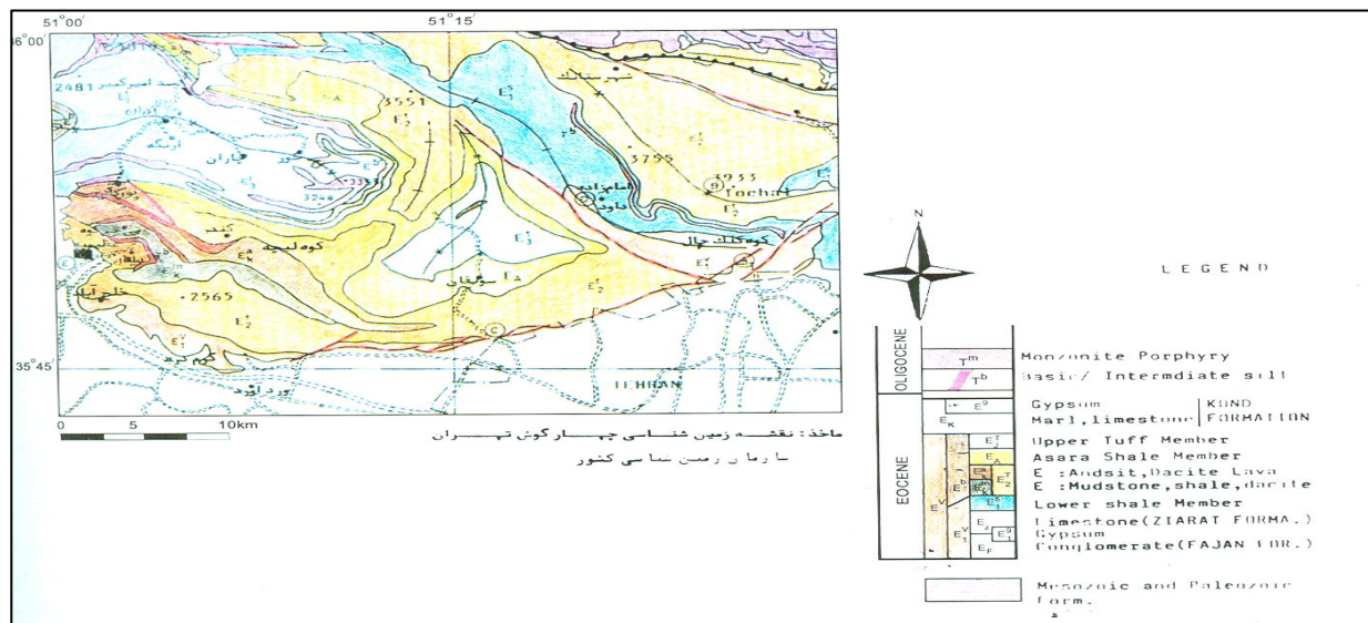
شکل ۱- نقشه زمین‌شناسی منطقه مورد مطالعه و موقعیت جغرافیایی مکان‌های اشاره شده در متن.
