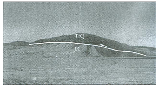
شکل ۲۰- از راندگی‌های کم شیب در مرز جنوبی پنجره آق‌دربند که سازند سرخ رنگ قره‌قیطان (TrQ) را بر روی طبقات تقریباً افقی سازند کشف رود (JK) رانده است. ۳/۵ کیلومتری شمال باختری روستای چشمه آزاد (نگاه به سمت باختر).
