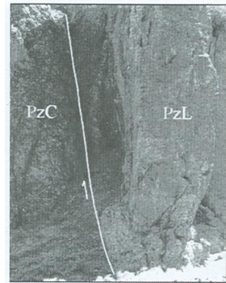
شکل ۹- گسل راندگی بین کنگلومرای پالتوزویک (PzC) در سمت چپ و مرمر پالتوزویک (PzL) در سمت راست. شیب این شکل گسلها به صورت ثانویه افزایش یافته و نزدیک به قائم شده است. ورودی دره شمالی معدن آق‌دربند (نگاه به سمت خاور).
