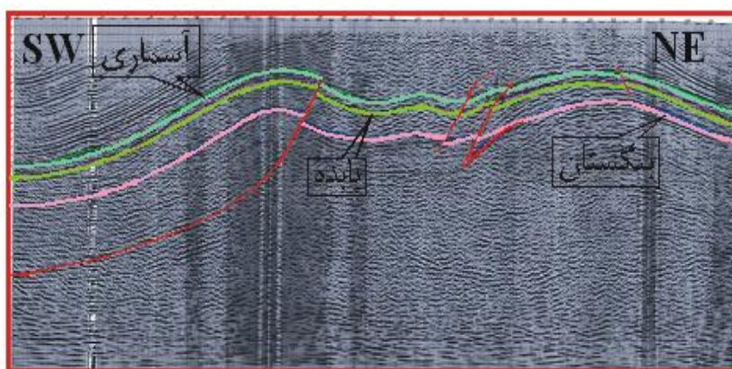
شکل ۱۲- تفسیر ساختاری نیمرخ بازتاب لرزه ای میدان های کرج و پارسی. موقعیت سر سازندهای مهم نشان داده شده است.
