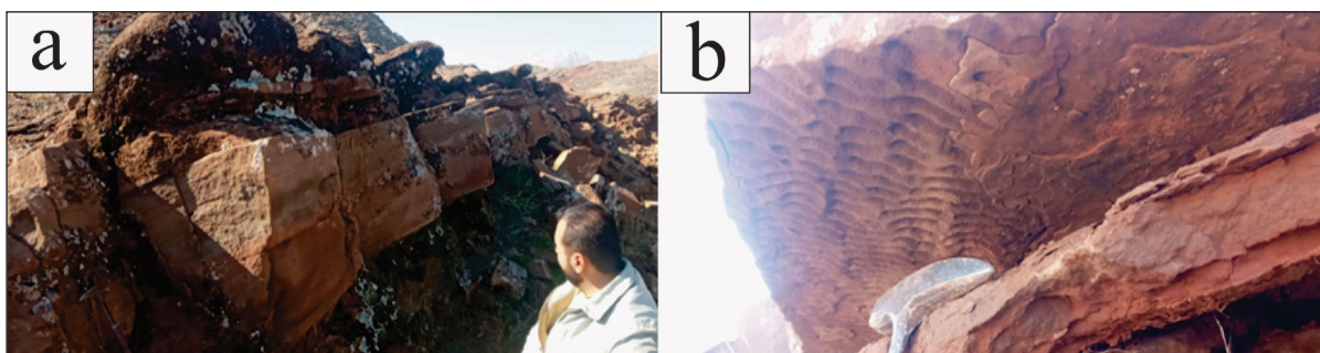
شکل ۱۸- (a) ماسه‌سنگ با ساخت افقی. (b) ماسه‌سنگ با ساخت افقی در زیر که بر روی آن ماسه موج‌نقشی قرار دارد. در زیر واحد ماسه‌سنگ افقی، ریپل کست (قالب موج‌نقش) شکل گرفته است.
