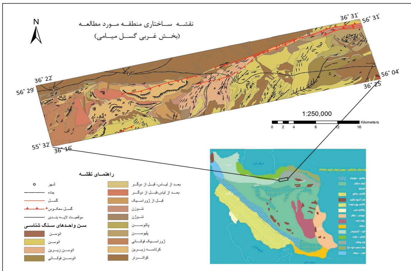
شکل ۱- نقشه زمین شناسی منطقه مورد مطالعه و موقعیت آن در نقشه پهنه بندی ساختاری نووی (۱۳۵۵).
