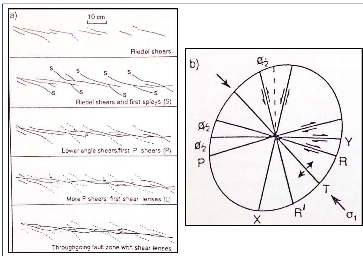
شکل ۹- (a) گسترش شکستگی های برشی ثانویه در نگاه نقشه (دید دوبعدی سطح) از آزمایش جعبه ماسه در گسل امتدادلغز راست گرد (برگرفته از (Naylor et al. (1986)؛ (b) پیچیدگی شکستگی های تئوری و آزمایشگاهی پیش بینی شده در طی برش ساده (برگرفته از (Bartlett et al. (1981).
