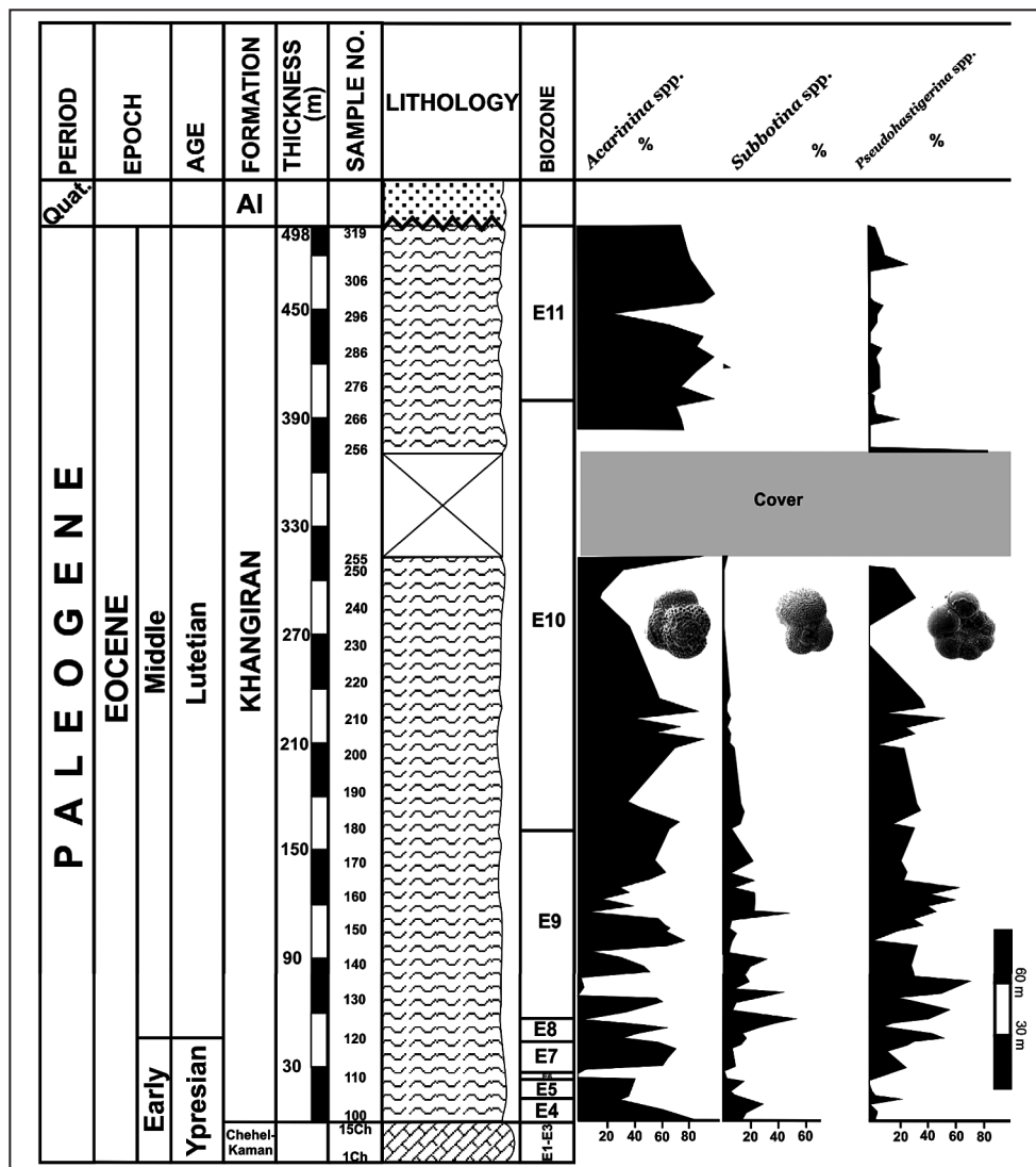
شکل ۶- نمودارهای درصد فراوانی نسبی ۳ جنس Subbotina , Pseudohastigerina و Acarinina در سازند خانگیران در برش مورد مطالعه.
