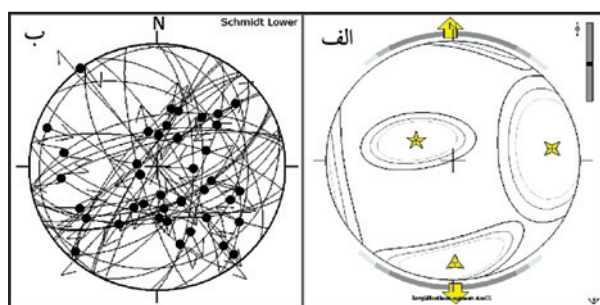
شکل ۸- نتایج تحلیل داده‌های اندازه‌گیری شده صحرایی درپاره شمالی. توضیحات این شکل با شکل ۶ یکسان است.
