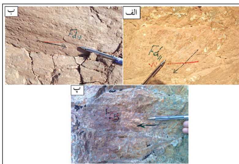
شکل ۱۱- نمونه‌ای از تصاویر صحرایی اندازه‌گیری شده گسل - خش در پاره شمالی. موقعیت صفحه و خش در هر یک از صفحات الف، ب و پ به ترتیب عبارتند از: الف) 63/046, 38/340؛ ب) 72/224, 18/140؛ پ) 90/053, 00/323.
