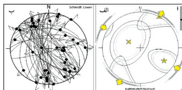
شکل ۱۴- نتایج تحلیل داده‌های اندازه‌گیری شده صحرایی مربوط به رژیم تنش امتدادلغزی در پاره میانی، توضیحات این شکل با شکل ۶ یکسان است.
