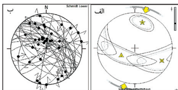
شکل ۱۳- نتایج تحلیل داده‌های اندازه‌گیری شده صحرایی مربوط به رژیم تنش فشاری در پاره میانی، توضیحات این شکل با شکل ۶ یکسان است.
