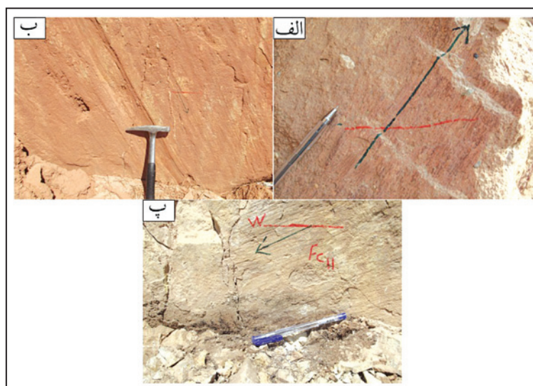
شکل ۱۰- نمونه‌ای از تصاویر صحرایی اندازه‌گیری شده گسل - خش در پاره میانی. موقعیت صفحه و خش در هر یک از صفحات الف، ب و پ به ترتیب عبارتند از: الف) 59/35, 43/049؛ ب) 68/045, 57/098؛ پ) 57/012, 30/304.
