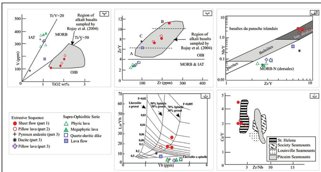
شکل ۸- نمودارهای گویای تعادل کالک و شوشنیتی روانه صفحه‌ای و گدازه‌های بخش‌های زیرین و میانی سکانس خروجی. الف) نمودار نسبت‌های Zr/Y به Nb/Y (Fitton & Godard, 2004; Brahic et al., 2006) (ب) نمودار نسبت Zr/Y به Zr (بازالت‌های جزایر اقیانوسی از تولیت‌های جزایر کمائی و مورب تفکیک شده‌اند. در این نمودار قلمروی الکالی بازالت‌ها بر اساس داده‌های Rojay et al. (2004) رسم شده است، (پ) نمودار نسبت V به TiO_2 که در آن قلمروی الکالی بازالت‌های جزایر اقیانوسی از تولیت جزایر کمائی و مورب تفکیک شده است (نقل از Shervais, 1982)، (ت) نمودار نسبت Ce/Y به Zr/Nb (نقل از Frey & Clague, 1983)، که آلکالی بازالت‌های بخش‌های زیرین و میانی توالی خروجی، با سی‌مونت‌های مختلف در اقیانوس آرام و جزیره سنت هلن در اقیانوس اطلس مقایسه شد، (ث) نمودار تغییرات Yb به La/Yb و (به نقل از Legendre et al., 2006; Blais et al., 2007) درجه‌های متفاوت ذوب بخشی نشان داده شد.
