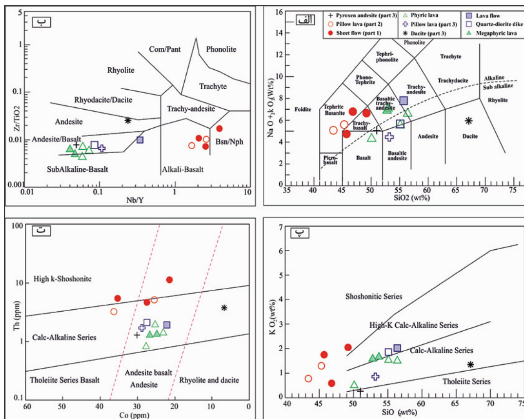
شکل ۴- الف) نمودار نامگذاری \text{SiO}_2 به \text{Na}_2\text{O}+\text{K}_2\text{O} ، پیشنهادی (Le Bas et al. 1986) و ب) نمودار نسبت \text{Nb/Y} به \text{Zr/TiO}_2 ، پیشنهادی (Winchester & Floyd 1976) و پ) نمودار متمایزکننده سری‌های ماگمایی، نسبت \text{SiO}_2 به \text{K}_2\text{O} ، پیشنهادی (Peccerillo & Taylor 1976) و ت) نمودار تعیین سری ماگمایی بر اساس نسبت \text{Th} به \text{Co} ، پیشنهادی (Hastie et al. 2007) که در آن از عناصر با تحرک کمتر مانند \text{Th} و \text{Co} استفاده شده است.
