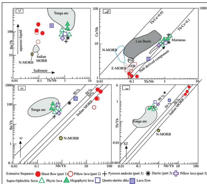
شکل ۷-الف) نمودار نسبت Th/Nb به Ce/Nb (نقل از Saunders and Tarney, 1984) که در آن نمونه‌های بخش بالایی توالی خروجی و سری سوپراافیولیتی با مقادیر بالاتر از (Th/Ce = 0.1) در محدوده کمان ماریان واقع شده‌اند. (ب) نمودار نسبت‌های Ba/Th به Th/Nb (نقل از Tian et al., 2008) که نشان می‌دهد که مذاب حاصل از ذوب بخشی رسوبات بالای صفحه فرورونده در ژنز توالی خروجی و سری سوپراافیولیتی مورد مطالعه ناچیز بوده، در عوض نقش سیالات آبدار آشکارتر است. (پ) نمودار نسبت‌های Th/Yb و Nb/Yb که می‌توان مقدار ترکیبات فرورانش (Subduction component) افزوده شده بر گوه گوشته‌ای بالای صفحه فرورونده را حدس زد. از داده‌های ژئوشیمیایی اقیانوس هند (Indian MORB) به‌عنوان شاخصی برای تشخیص افیولیت‌های نوع مورب (MORB) و داده‌های ژئوشیمیایی کمان Tonga به‌عنوان معیاری برای تمایز مناطق کمائی (که در آنها نقش سیالات در ژنز ماگما آشکارتر است) استفاده شد (Pearce & Peate, 1995; Pearce et al., 2005). (پ) نمودار نسبت Nb/Yb به Ba/Yb ، که نشان می‌دهد که میزان مشارکت عنصر Ba در سیال‌های برخاسته از صفحه فرورونده از حدود ۳۰ درصد در نمونه‌های بخش‌های زیرین و میانی توالی خروجی تا بیش از ۹۰ درصد در نمونه‌های بخش بالایی توالی خروجی و گدازه‌های سری سوپراافیولیتی متغیر است. نمودارهای ب، پ و ت از Tian et al. (2008) برگرفته شده‌اند.
