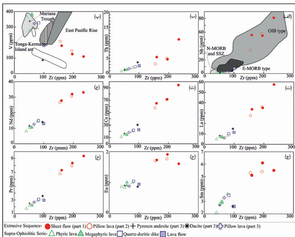
شکل ۵- نمودارهای دو گانه بر حسب نسبت Zr به عناصر فرعی و کمیاب V، Th، Nb، La، Ce، Nd، Sm، Eu، Pr، را نشان داده است. قلمروهای تعریف شده در شکل ۵-الف، از Miyashita et al. (2003) و قلمروهای شکل ۵-ب از Dubois-Cote et al. (2005) برگرفته شده‌اند.
