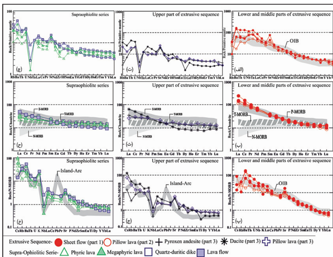
شکل ۶- نمودارهای عنکبوتی بهنجار شده با مقادیر استاندارد کندریت و گشته اولیه که بر اساس داده‌های Sun and Macdonough (1989) رسم شده‌اند. محدوده‌های میانگین N-MORB، T-MORB، P-MORB، back arc بر اساس داده‌های Nicholson et al. (2000) رسم شده‌اند. و fore arc محدوده‌های میانگین Sun and Macdonough (1989) بر اساس داده‌های
