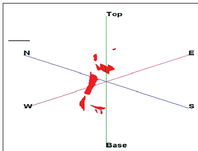
شکل ۲- تفکیک رگه و رگچه‌های حاوی کانی‌سازی طلا در کانسار قفله.
