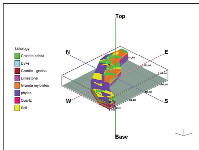
شکل ۳- مدل کلی سنگ‌شناسی کانسار طلای قفله.
