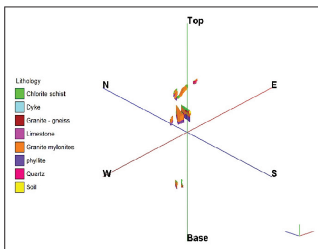
شکل ۴- مدل سنگ‌شناسی میزبان رگه‌های حاوی کانی‌سازی طلا در کانسار قفله.
