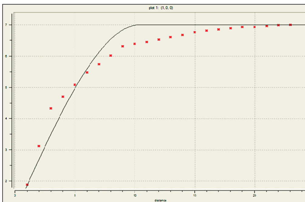
شکل ۵- واریوگرام عنصر طلا در کانسار قفله.
