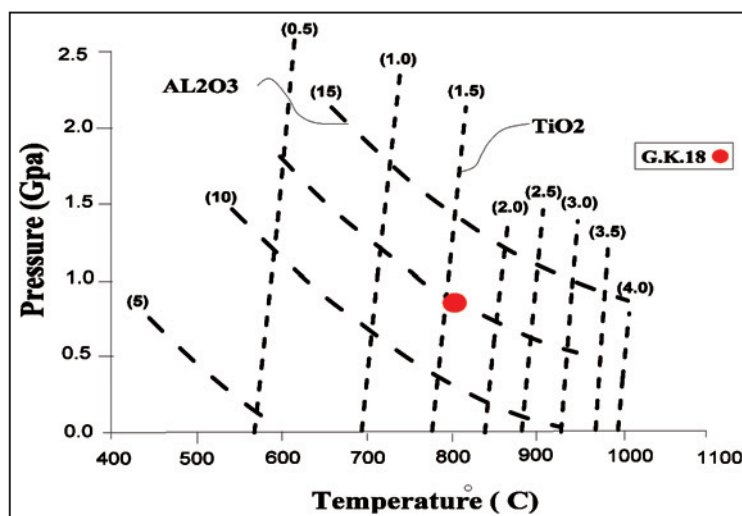
شکل ۱۳- با استفاده از دما فشارسنجی بر اساس اکسیدهای آلومینیم و تیتانیم موجود در تکت کانی آمفیبول (Ernest & Liu, 1998)، دمایی حدود ۸۰۰ درجه سانتی گراد در فشاری معادل ۷ تا ۸ کیلو بار برای سنگ های گابرویی ارزیابی می شود.
