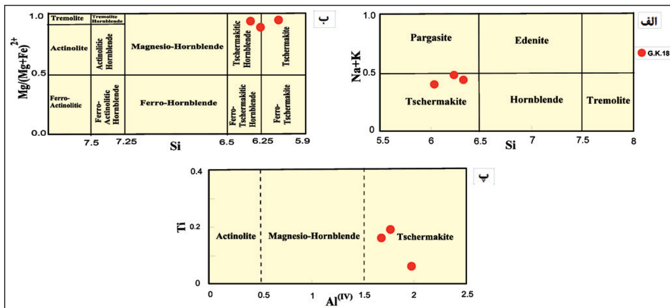
شکل ۱۰- الف) آمفیبول‌های تجزیه شده نمونه مافیک (G.K.18) در نمودار (Na+K)-Si (Leak et al., 1997) از نوع چرمایت است؛ ب) این کانی‌ها با در نظر گرفتن نسبت کاتیونی Mg/(Mg+Fe^{2+}) در برابر Si در محدوده چرمایت و هورنبلند چرمایتی قرار گرفته‌اند؛ پ) ترکیب شیمیایی آمفیبول‌ها در نمودار مقادیر کاتیونی Ti در برابر Al تراهدرال سایت نیز از نوع چرمایت مشخص می‌شوند.
