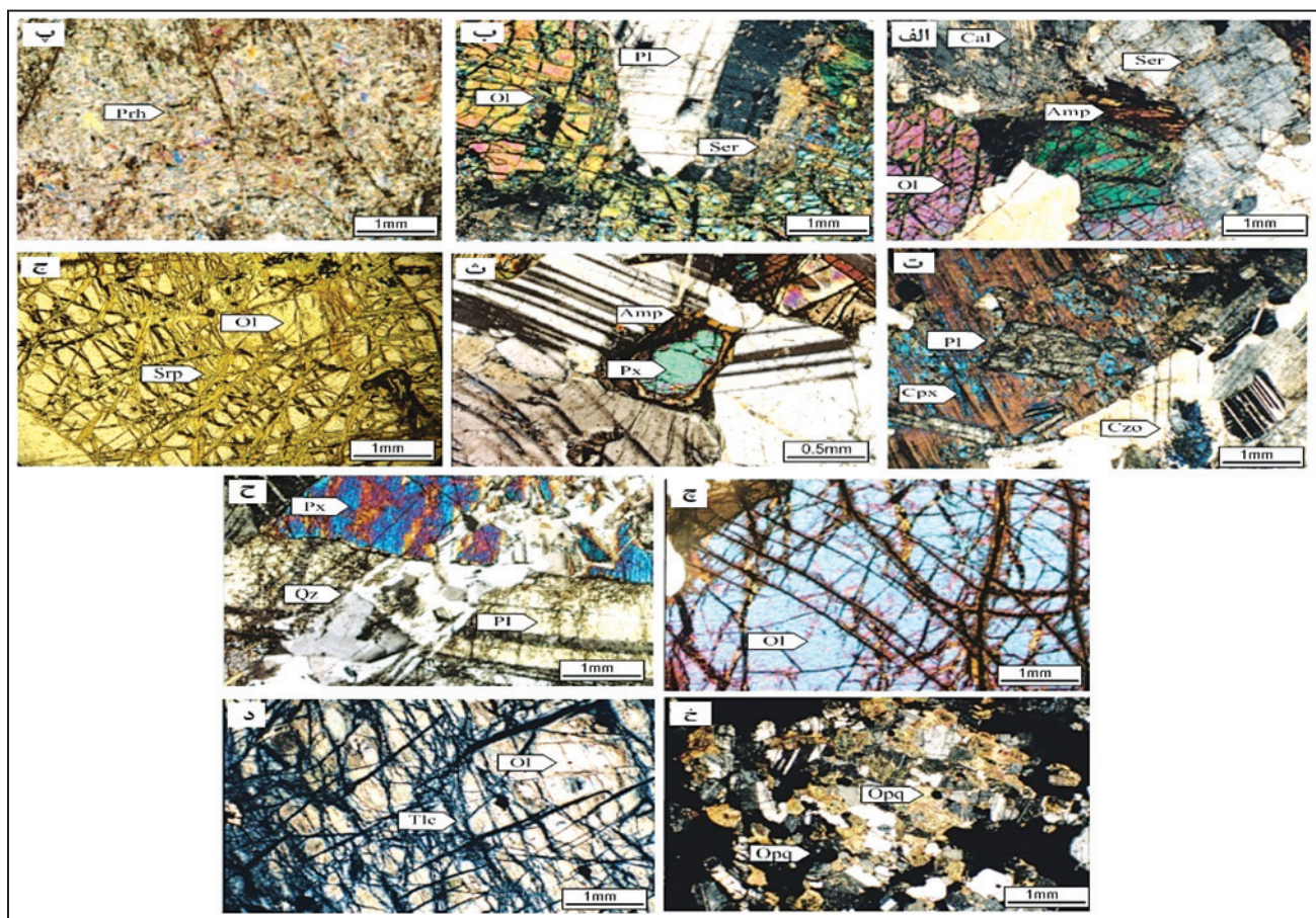
شکل ۲- تصاویر سنگ نگاری نمونه‌های مافیک (گابرو) و اولترامافیک مورد بررسی (XPL) به استثنای تصویر (ج، PPL)؛ الف) کلسیت و سریسیت حاصل از دگرسانی پلاژیو کلازها؛ ب) درشت‌بلور پلاژیو کلاز که از حاشیه سریسیتی شده است؛ پ) پره‌نیت حاصل از دگرسانی پلاژیو کلاز آنورتیت؛ ت) بلورهای پلاژیو کلاز که با جهت یافتگی اتفاقی به وسیله کانی‌های پیروکسن احاطه شده‌اند و کلاینوزونیزیت‌هایی که از دگرسانی پلاژیو کلازها حاصل شده‌اند؛ ث) بلور پیروکسن که از حاشیه به اورالیت دگرسان شده است؛ ج) درشت‌بلور الیون دگرسان‌شده به کانی‌های رشته‌ای مانند سرپانتین؛ چ) درشت‌بلور الیون که درون شکستگی‌های آن ایدنگزیت دیده می‌شود؛ ح) رگه ثانویه کوارتز که از پیروکسن و پلاژیو کلاز عبور کرده است؛ خ) کانی‌های کدر موجود درون بلورها و متن سنگ؛ د) درشت‌بلور الیون دگرسان‌شده به کانی‌های رشته‌ای مانند تالک. نشانه‌ها: پلاژیو کلاز = Pl؛ پیروکسن = Px؛ کلاینوپیروکسن = Opq؛ کلسیت = Cal؛ سریسیت = Ser؛ تالک = Tlc؛ پره‌نیت = Prh؛ کلاینوزونیزیت = Czo؛ کوارتز = Qz؛ کدر = Opq.
