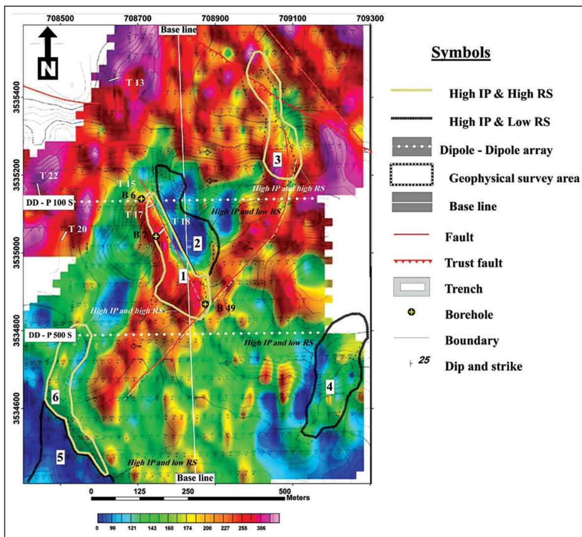
شکل ۷ - نقشه مقاومت ویژه ظاهری محدوده مطالعاتی با تغییرات (محمدی و یژه، ۱۳۹۰)
