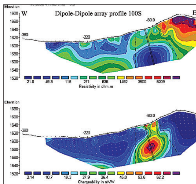
شکل ۸ - مقاطع دو بعدی مقاومت ویژه و بارپذیری، نیمرخ 100S (محمدی و یژه، ۱۳۹۰)
