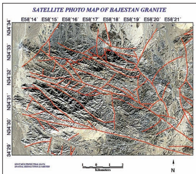
شکل ۶- رسم خطواره‌های اصلی به صورت وکتور بر روی داده SPOT.
