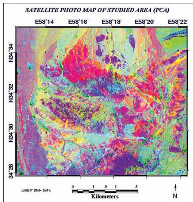
شکل ۸- تصویر حاصل از روش PCA انتخاب ۴ بانندی، حاصل از ترکیب RGB = PCband3(1.3.4.5), PCband1(1.3.4.5), -PC4(1.3.5.7) .
