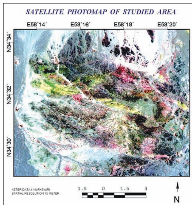
شکل ۹- تصویر حاصل ترکیب بانندی RGB: 468 با استفاده از داده‌های ASTER.
