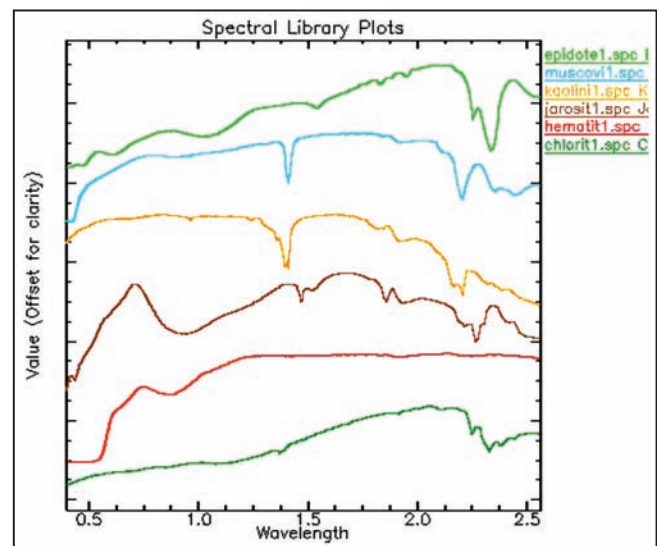
شکل ۱۱- نمودار طیفی کانی‌های کلریت، هماتیت، جاروسیت، کانولینیت، سیرسیت و اپیدوت (با استفاده از کتابخانه طیفی USGS).
