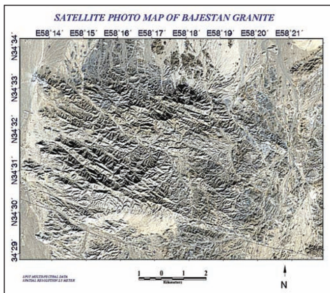
شکل ۴- تصویر محدوده مورد مطالعه با استفاده از پردازش داده‌های SPOT و اعمال فیلتر High Pass نوع 11*11 Sharpen برای بارزسازی خطواره‌ها.
