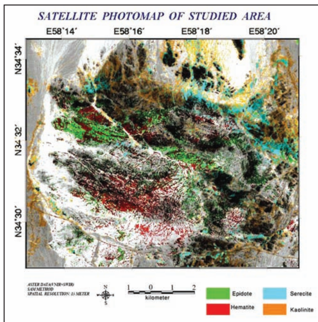
شکل ۱۲- تصویر حاصل از پردازش داده ASTER به روش SAM برای کانی‌های اپیدوت، سیرسیت، هماتیت و کانولینیت.
