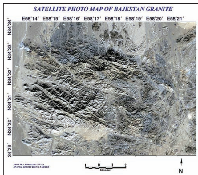
شکل ۳- تصویر محدوده مورد مطالعه با استفاده از پردازش داده‌های SPOT با هدف تفکیک مرز واحدهای زمین‌شناسی.
