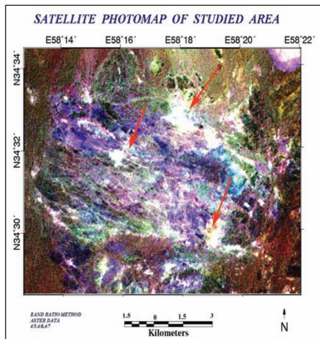
شکل ۱۰- تصویر حاصل از روش نسبت بانندی به صورت RGB: 4/5, 4/6, 4/7 ، بر روی داده ASTER، مناطق دارای دگرسانی بارز، با فلش مشخص شده است.
