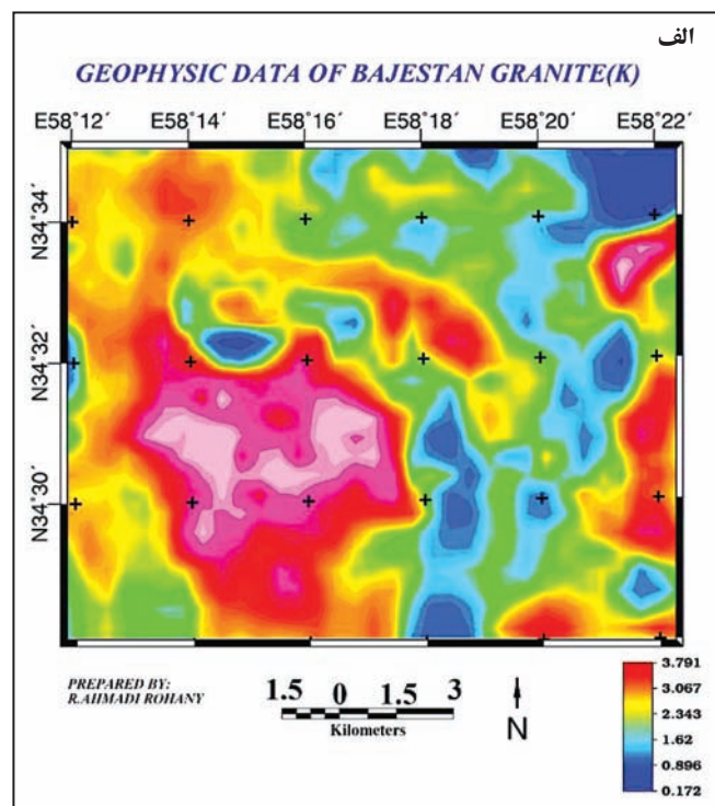
شکل ۱۳- پردازش داده‌های ژئوفیزیک هوایی: الف) شمارش پتاسیم (K)؛ ب) شمارش توریم (Th).
