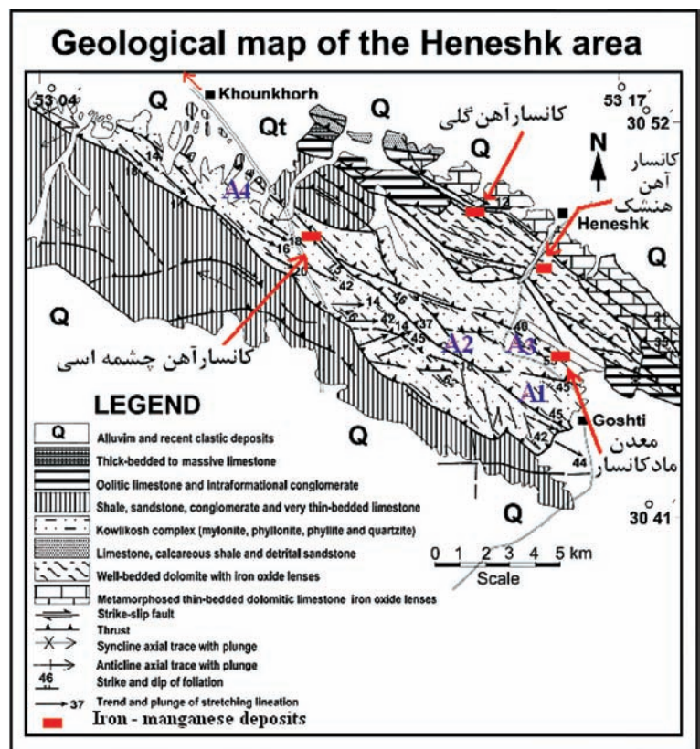
شکل ۶- پهنه برشی هنشک و موقعیت کانسارهای آهن‌مگنزدار گوشتی- هنشک، گلی و چشمه اسی (Sarkarinejad & Azizi, 2008).
