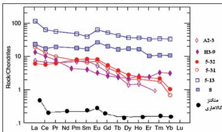
شکل ۲۳- الگوی عناصر خاکی کمیاب کانسارهای مورد مطالعه (به‌ویژه نمونه ۵ تا ۱۳) و مقایسه آن با الگوی کاندزایی منگنز میدان کالاهاری (Cornell & Schutte, 1995) که خاستگاه آتشفشانی-بروندمی دارد (جایگاه نمونه‌ها و معادن مربوط در جدول ۲ ارائه شده است).
