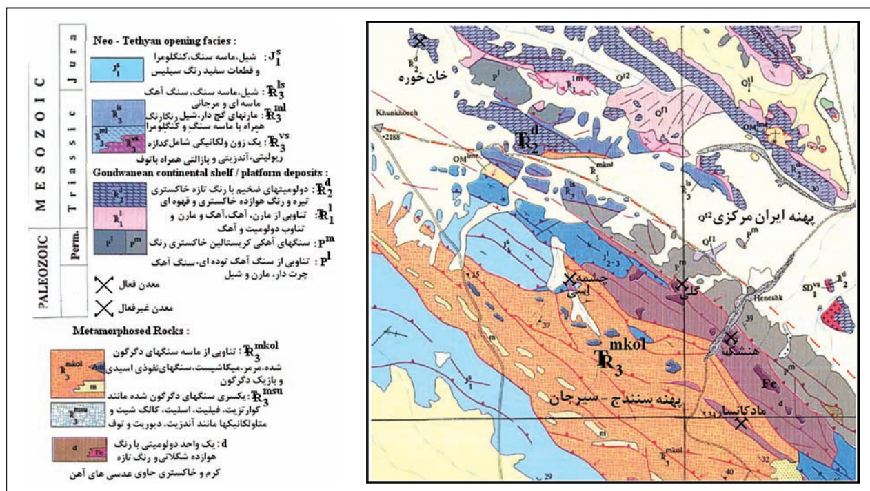
شکل ۲- بخشی از نقشه ۱:۱۰۰۰۰۰ دهیید که دو پهنه ایران مرکزی و سندج- سیرجان را در بر دارد. در این نقشه دولومیت‌های تریاس میانی ( TR_2^d ) از ایران مرکزی روی واحدهای تریاس بالایی ( TR_3^{mkl} ) کمپلکس دگرگونی کولی‌کش) در سندج- سیرجان رانده شده و دولومیت‌های دارای عدسی‌های آهن (d) را تشکیل داده‌اند (شهیدی، ۱۳۷۴). معدن آهن منگنزدار خان‌خوره (بخش شمال باختری نقشه) در دولومیت‌های تریاس میانی ( TR_2^d ) در پهنه ایران مرکزی و معادن آهن منگنزدار گوشتی- هنشک (مادکانسار)، چشمه اسی و گلی در دولومیت‌های دارای عدسی آهن (d) در پهنه سندج- سیرجان قرار دارند.
