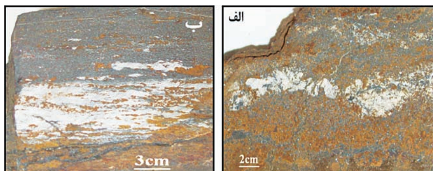
شکل ۱۴- الف و ب) نمونه دستی از دولومیت حامل آهن منگنزدار غنی از سیلیس با بافت لامینه یا نواری که در آن نوارهای تیره (هماتیت و مگنتیت) و نوارهای روشن سیلیس هستند، معدن مادکانسار.
