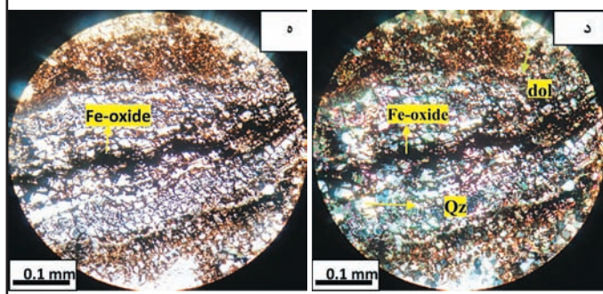
شکل ۱۵- الف) چین خوردگی عدسی‌های آهن منگنزدار همراه با دولومیت در مقیاس رخنمون؛ ب) نمونه دستی از دولومیت دارای آهن منگنزدار غنی از سیلیس، در کانسار چشمه اسی؛ ج) بخش بزرگ شده شکل ب که در آن لامینه‌های اکسید آهن منگنزدار چین خورده‌اند؛ د و ه) چین خوردگی Convolute مانند در لامینه‌های ماده معدنی، هماتیت- مگنتیت (نوارهای تیره) همراه با دولومیت‌ها (dol) و کوارتز (نوارهای روشن) در کانسار چشمه اسی؛ د) نورمقاطع؛ ه) نور ساده.
