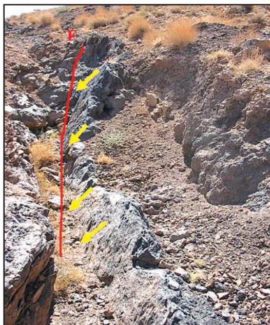
شکل ۹- گسل عادی جوان که باعث تمرکز ماده معدنی، در کانسار گلی شده است، پیکان‌ها جهت حرکت قطعه فرادیواره را نشان می‌دهند.
