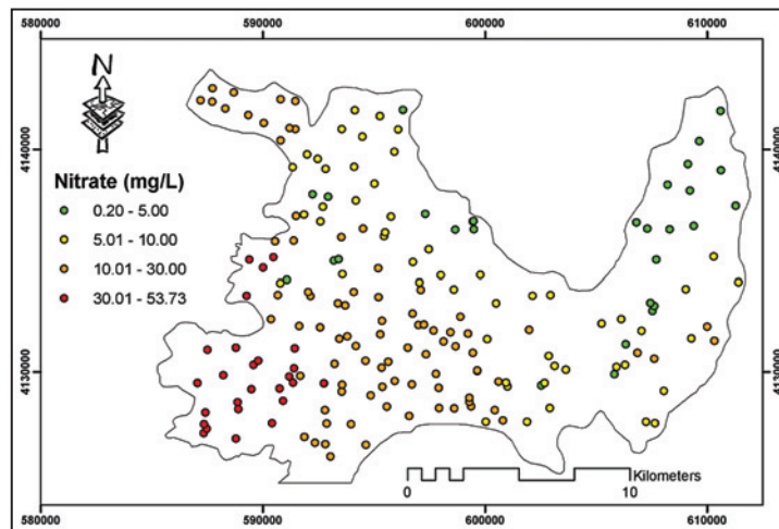
شکل ۴- غلظت نیترات در نقاط مختلف منطقه مورد مطالعه.
