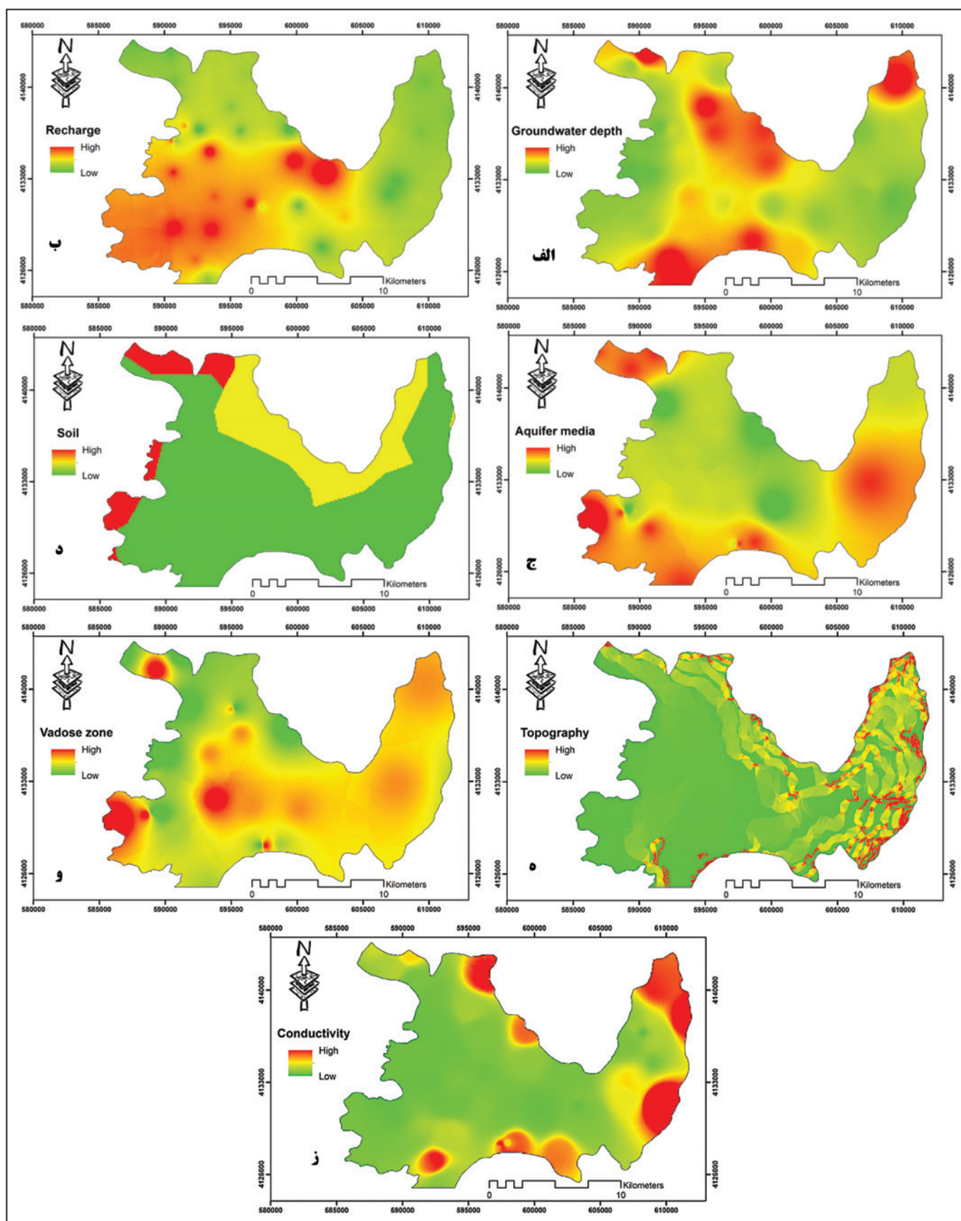
شکل ۳- نقشه پهنه‌بندی پارامترهای دراستیک؛ الف) ژرفای آب زیرزمینی؛ ب) تغذیه؛ ج) محیط آبخوان؛ د) محیط خاک؛ ه) شیب سطح زمین؛ و) زون غیراشباع؛ ز) هدایت هیدرولیکی.
