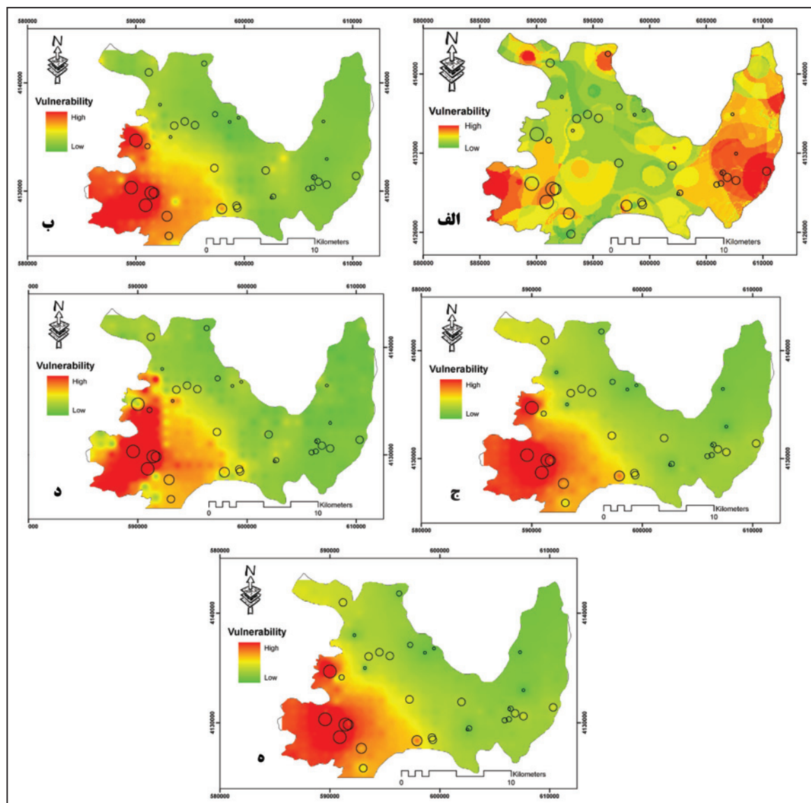
شکل ۵- نقشه آسیب‌پذیری آب زیرزمینی منطقه مورد مطالعه با استفاده از روش‌های مختلف؛ الف) مدل دراستیک اولیه؛ ب) مدل ANN؛ ج) مدل SFL؛ د) مدل MFL؛ ه) مدل نروفازی.
