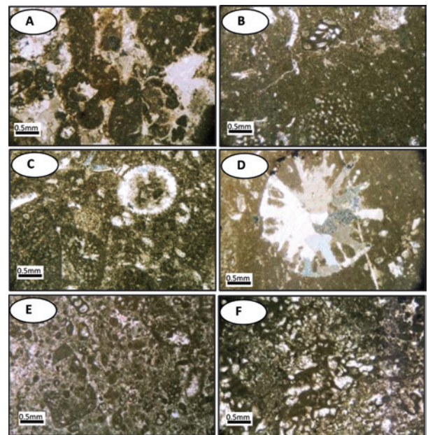
شکل ۴- ریزرخساره‌های محیط‌های میان‌کشدی و لاگون سازند داریان در برش‌های مورد مطالعه. (A) رخساره اینتراکلاست گرینستون که مشخص کننده محیط کانال‌های کشدی است. برش کوه سیاه، نمونه شماره ۷۳، نور پلاریزه. (B) ریزرخساره بنتیک فرامینیفرا و کستون، برش کوه سیاه، نمونه شماره ۶۴، نور پلاریزه. (C) ریزرخساره و کستون/پکستون داسی‌کلاداسه‌آ، پلویید، اربیتولین دار، برش کوه سیاه، نمونه شماره ۵۹، نور پلاریزه. (D) ریزرخساره اسکلاکتینا فلوتستون، مربوط به محیط لاگون، برش کوه سیاه، نمونه شماره ۷۹، نور پلاریزه. (E) ریزرخساره بنتیک فرامینیفرا پلویید پکستون/گرینستون مربوط به زیر محیط پشته‌های ماسه‌ای، برش کوه سیاه، نمونه شماره ۲۳، نور پلاریزه. (F) ریزرخساره لیتوکودیوم باندستون، برش کوه سیاه، نمونه شماره ۲۴، نور پلاریزه.
