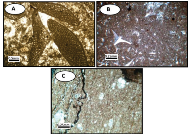
شکل ۷- ریزرخساره‌های سازند داریان در برش‌های مورد مطالعه. (A) ریزرخساره پلوئید، اربیتولین پکستون مربوط به دریای باز، برش کوه‌سیاه، نمونه شماره ۸۵، نور طبیعی. (B) وکستون با اجزای اسکلتی که در آن کرینویید پلاژیک کوماتولیدا مربوط به محیط دریای باز ژرف، برش کوه‌سیاه، نمونه شماره ۱۰۳، نور پلاریزه. (C) ریزرخساره مادستون / وکستون بایوکلاست‌های پلانکتون‌دار، برش چاه سبزه‌پوشان، ژرفای ۲۰-۶۲۱۵ فوتی، نور پلاریزه.
