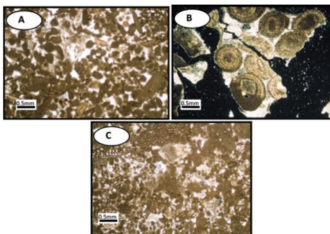
شکل ۵- ریزرخساره‌های محیط پشته‌های ماسه‌ای در برش‌های مورد مطالعه سازند داریان. (A) ریزرخساره پلویید اینتراکلاست گرینستون که در آن بیشتر پلوییدها از نوع پلت‌های سنگی است. برش کوه سیاه، نمونه شماره ۱۶، نور پلاریزه. (B) ریزرخساره بنتیک فرامینیفرا توید گرینستون با اتوئیدهای هم‌مرکز کم و بیش یک اندازه مشخص می‌شود. برش چاه سبزویشان، ژرفای ۸۵-۵۷۸۰ فوتی، نور پلاریزه. (C) ریزرخساره اینتراکلاست کریئوئید پکستون مربوط به بخش دریایی پشته‌های ماسه‌ای، برش کوه سیاه، نمونه شماره ۱۷، نور پلاریزه.
