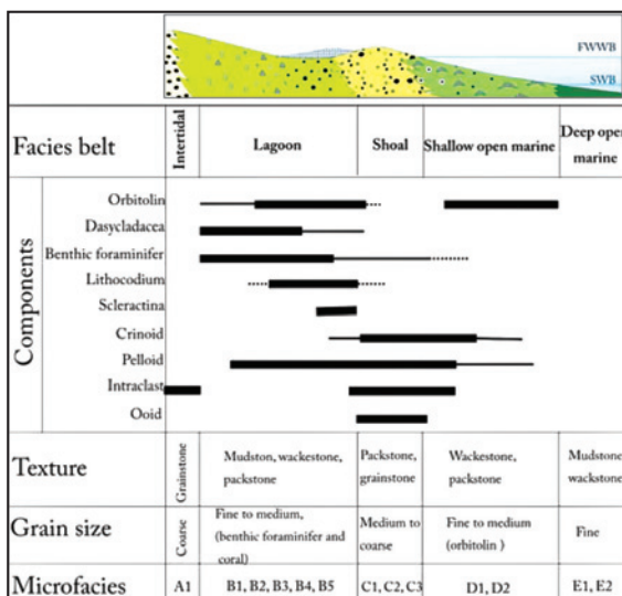
شکل ۹- پراکنندگی جانبی رخساره‌ها و اجزای اسکلتی و اجزای غیر اسکلتی در برش‌های مورد مطالعه سازند داریان.
