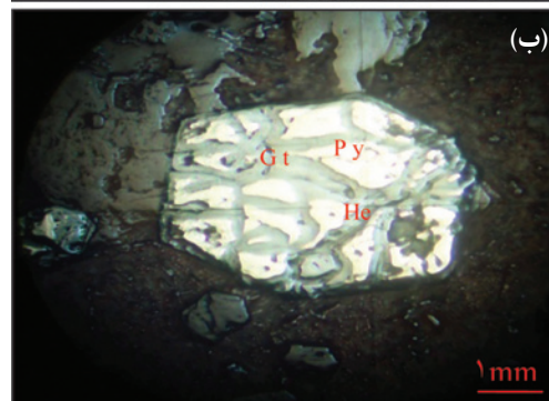
شکل ۸- الف) پیریت نسل اول که بسیار درشت دانه است و با چشم غیر مسلح به راحتی دیده می‌شود از حاشیه در حال تبدیل به گوئیتیت و هماتیت است و در بخش (ب) به شکل جزیره‌های در حال تبدیل به هماتیت و گوئیتیت است. (نور xpl).
