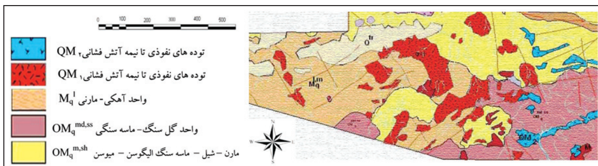
شکل ۲- نقشه زمین‌شناسی (توده‌های نفوذی که در بخش جنوبی واقع شده‌اند) منطقه شائق با مقیاس ۱:۵۰۰۰
