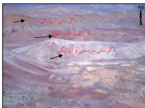
شکل ۴- دگرسانی آرتزلیک ، سریستیک و اکسیدهای آهن (هماتیت، گوتیت و لیمونیت) در توده‌های نفوذی که به دلیل شدت بالای دگرسانی بسیار درهم است.
