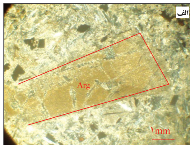
شکل ۵- الف) کانی‌های فلدسپار که به شدت دچار دگرسانی آرتزلیکی شده‌اند. ب) دگرسانی سریستی در فلدسپارها (نور شکل الف ppl و تصویر ب XPL).
