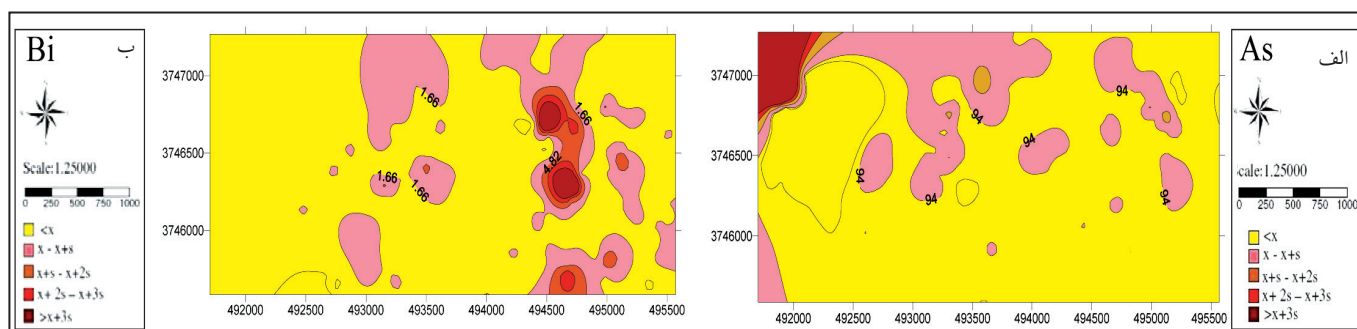
شکل ۱۶- نقشه بی‌هنجاری ژئوشیمیایی الف (آرسنیک و ب) بیسموت، در توده‌های نفوذی در منطقه جنوبی شائق.
