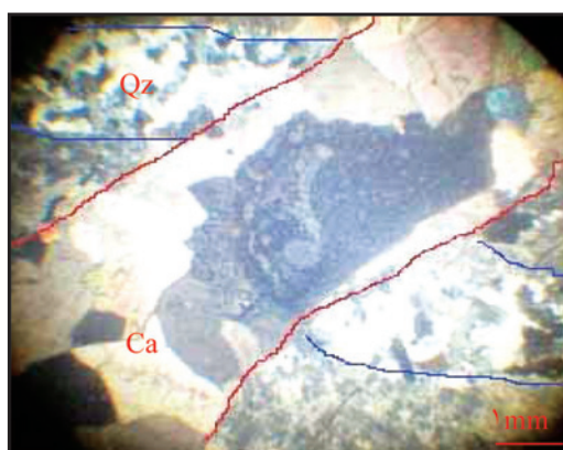
شکل ۷- رگه‌های کوارتز که توسط رگه‌های کربناتی قطع شده است (نور xpl).
