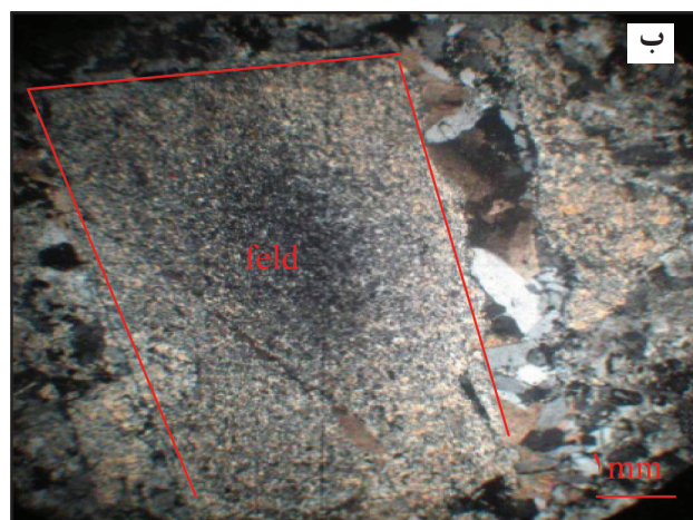
شکل ۵- الف) کانی‌های فلدسپار که به شدت دچار دگرسانی آرتزلیکی شده‌اند. ب) دگرسانی سریستی در فلدسپارها (نور شکل الف ppl و تصویر ب XPL).
