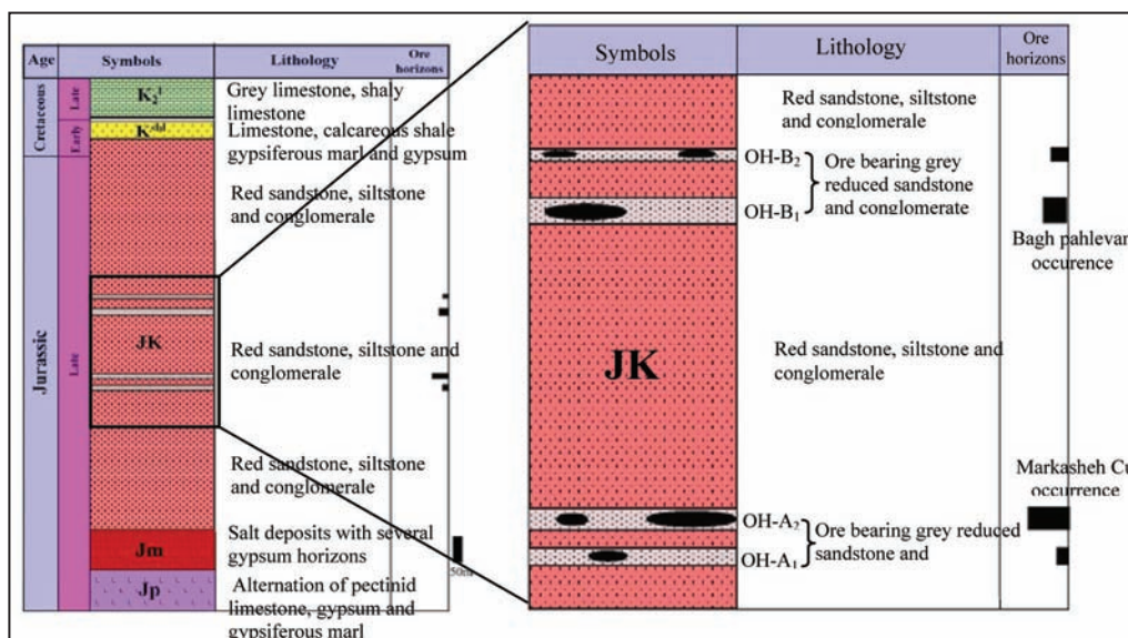
شکل ۳- ستون چینه‌شناسی عمومی از منطقه معدنی مارکشه و موقعیت افق‌های احیایی کاندار در آن.
