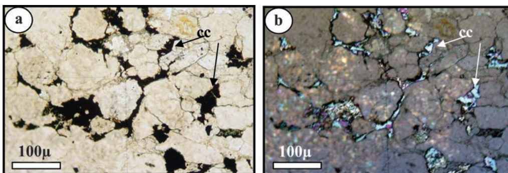
شکل ۱۳- نمایی از بافت سیمان میان دانه‌ای یا Impregnation در بین دانه‌های آواری سنگ میزبان در پهنه احیایی کانه‌زایی شده که در آن کالکوسیت (cc) به صورت سیمان بین دانه‌های آواری را پر کرده است. (a) در نور عبوری و (b) در نور بازتابی
