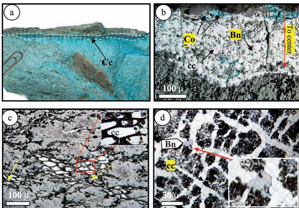
شکل ۱۲- (a) جانیشینی فسیل گیاهی توسط کالکوسیت (a) کانی کالکوسیت که به صورت یک نوار باریک از حاشیه جانیشین فسیل گیاهی شده است. (b) جانیشینی سولفیدهای مس (کالکوسیت، کولیت و بقایایی از بورنیت) از حاشیه به سمت مرکز فسیل گیاهی (نور ان بازتابی در محیط Oil). (c) جانیشینی سلولار در فسیل‌های گیاهی توسط کالکوسیت. (d) جانیشینی آوندهای فسیل گیاهی توسط سولفیدهای مس. cc= کالکوسیت، Bn= بورنیت، Co= کولیت.
