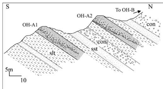
شکل ۶- مقطع عرضی از افق‌های اصلی کاندار OH-A و OH-B و موقعیت زیر افق‌های آن نسبت به یکدیگر. slt - سیلتستون. sst - ماسه‌سنگ. con - کنگلومرا.
