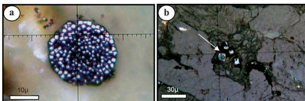
شکل ۱۱- (a) نمایی از پیریت فراموئیدال که در مرحله دیاژنز اولیه و پس از ته‌نشست ژل سولفیدی از آن متبلور شده است (نور بازتابی در محیط Oil). (b) پیریت دیاژنتیک خودشکل. هر دو نوع پیریت به صورت پراکنده در متن سنگ دیده می‌شوند.
