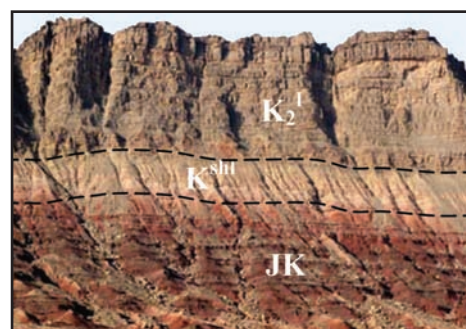
شکل ۴- نمای عمومی از لایه‌های سرخ گره‌دو (JK) که توسط واحدهای سنگی مارن گچ‌دار (K shl ) و آهک‌های سبتر لایه کرتاسه (K 2 1 ) پوشیده می‌شود.
