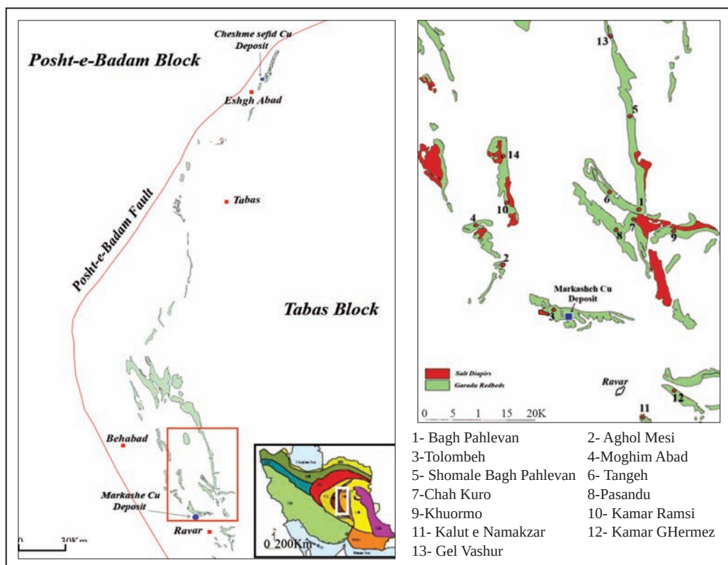
شکل ۱- گسترش سازند سرخ گره‌دو و کانی‌سازی مس در پهنه مس رسوبی راور- طبس- عشق‌آباد و پراکنندگی رخدادهای اندیس‌های مس در آن در بلوک طبس. به نحوه گسترش و همراهی گنبد‌های نمک به سن ژوراسیک بالا با سازند سرخ گره‌دو توجه شود.
