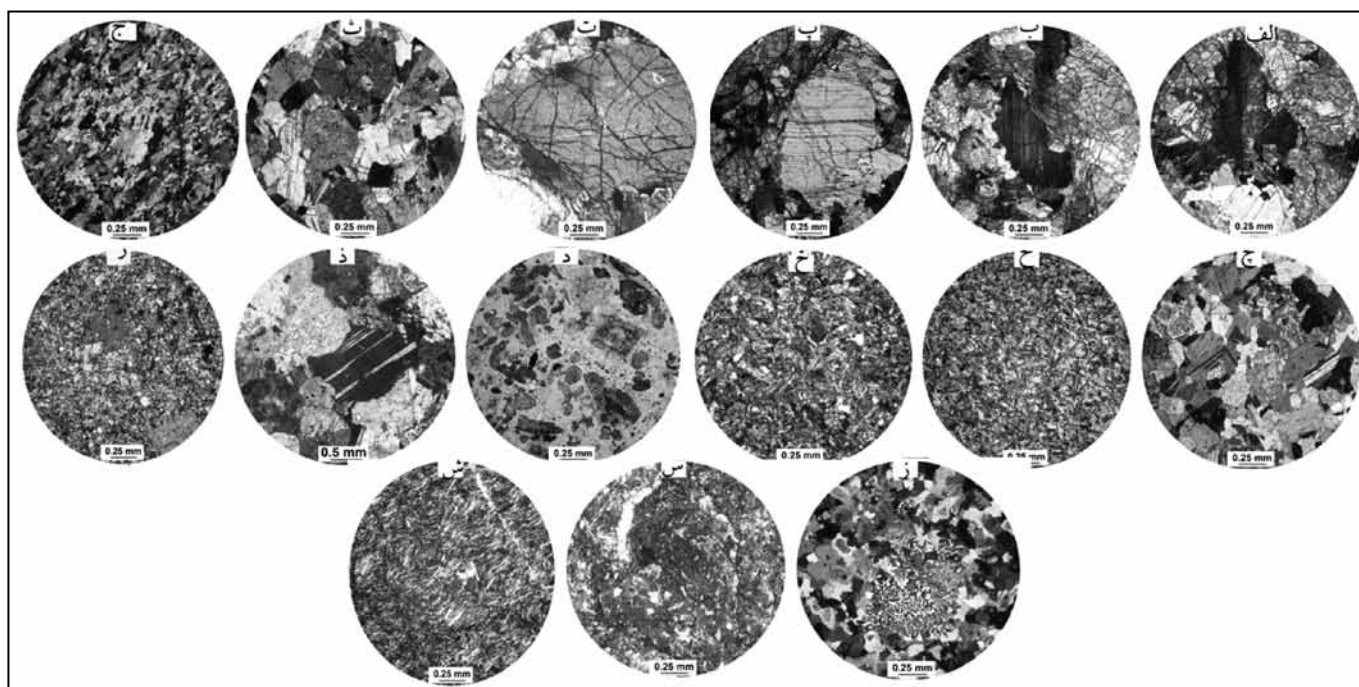
شکل ۵- تصاویر میکروسکوپی انتخابی شامل الف) الیون با ساختار داخلی کینک در هارزبورژیت با دگرشکلی گوشته‌ای، ب) نوارهای نازک دیوپسید در درون آتستاتیت، پ) بلور درشت نادگرشکل دیوپسید در لرزولیت، ت) بلورهای ریز الیون فاقد ساختار کینک در درون ارتوپروکسن بلورهای الیون دگرشکل در پایین مقطع دیده می‌شوند، ث) پیروکسن، گابرو، ج) هورنبلاند گابرو، چ) ارتوپروکسن در الیون-گابرو، ح) دیاباز ریزبلور، خ) دیاباز دارای بلورهای ریز کوارتز، د) کوارتز دیوریت آمفیبول دار، ذ) پگماتیت گابرو، ر) پلاژیوگرانیت با بافت فیریک و خمیره ریزبلور، ترونجیت با بافت میکروپگماتیت گرافیک، س) جاننشینی شیشه آتشفشانی با اسمکتیت زیتونی رنگ، ش) بافت میکروولیتیک جریان در صفحه‌ای.
