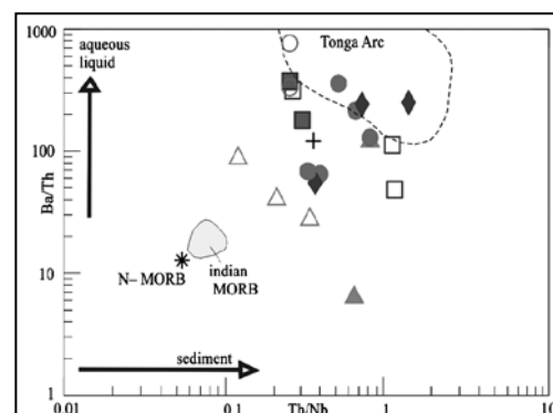
شکل ۹- موقعیت تجزیه‌های منطقه و تأثیر بیشتر سیال‌ها و نقش کمتر رسوبات در ژئز افیولیت کهدونیه. داده‌ها از Tian et al. (2008) و منابع آن استفاده شده است.
