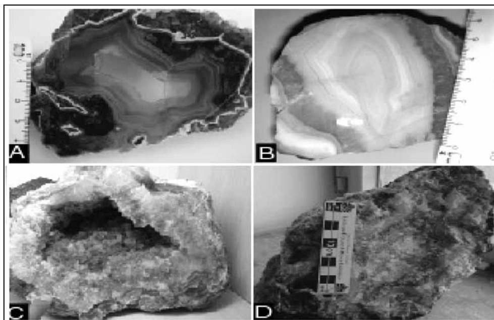
شکل ۷- (A) عقیق عسلی (B) عقیق طوسی (C) آمیتیسیت (D) عقیق آبی با رگه کوارتز قرمز
