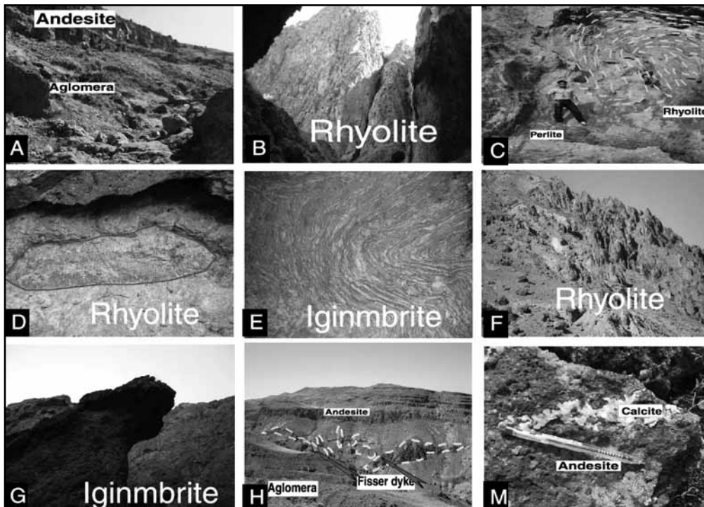
شکل ۵- A) نمایی از آگلومراهای منطقه B) ساخت تافونی (لانه کبوتری) در رپولیت‌های منطقه C) فرسایش و ساخت جریان‌های شدید در رپولیت‌ها D) فرسایش پوست پیازی E) ساخت جریان‌های شدید در ایگنمبریت‌ها F) مخروط‌های رپولیتی G) اشکال مختلف در ایگنمبریت‌ها H) فیشر دایک‌ها در درون آگلومراها و برش‌های آتشفشانی M) ساخت حفره‌های در آندزیت‌ها که با کلسیت و سیلیس پر شده‌اند.
