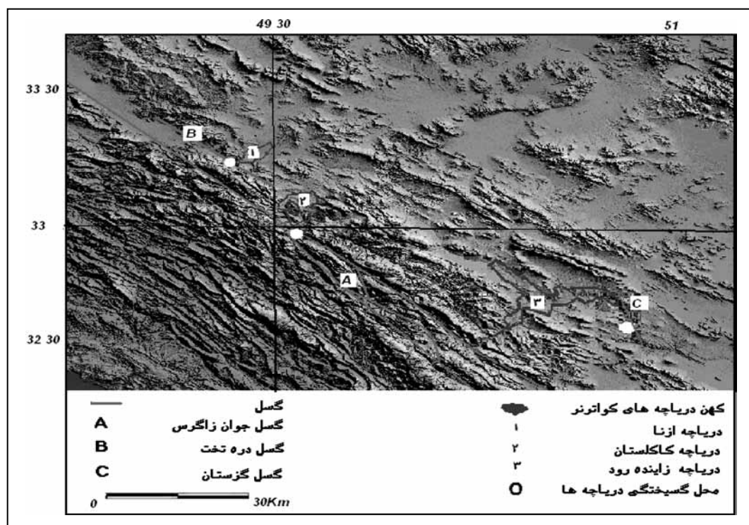
شکل ۶- بازسازی محدوده کهن دریاچه‌های کواترنری در پشت گسل جوان زاگرس.
