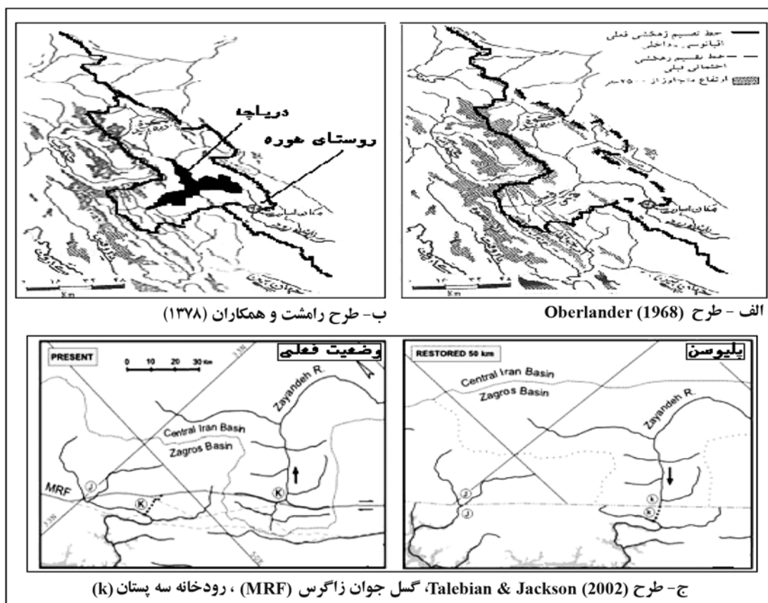
شکل ۱- سه دیدگاه در مورد وضعیت سرشاخه‌های زاینده‌رود الف) طرح (1968) Oberlander، ب) طرح رامشت و همکاران (۱۳۷۸)، ج) طرح (2002) Talebian & Jackson.
