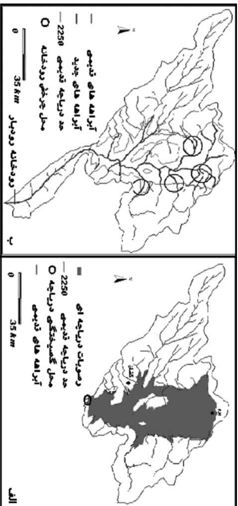
شکل ۵- وضعیت شبکه آبراهه‌ها در حوضه کاکستان، الف) - در زمان وجود دریاچه، ب) - پس از گسیختگی دریاچه.
