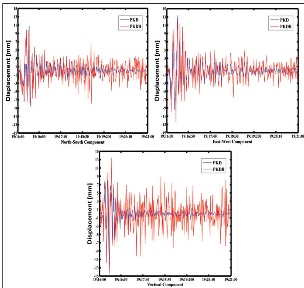
شکل ۶- مقایسه داده های لرزه نگاری و GPS آهنگ بالا برای ایستگاه PKD و PKDB
