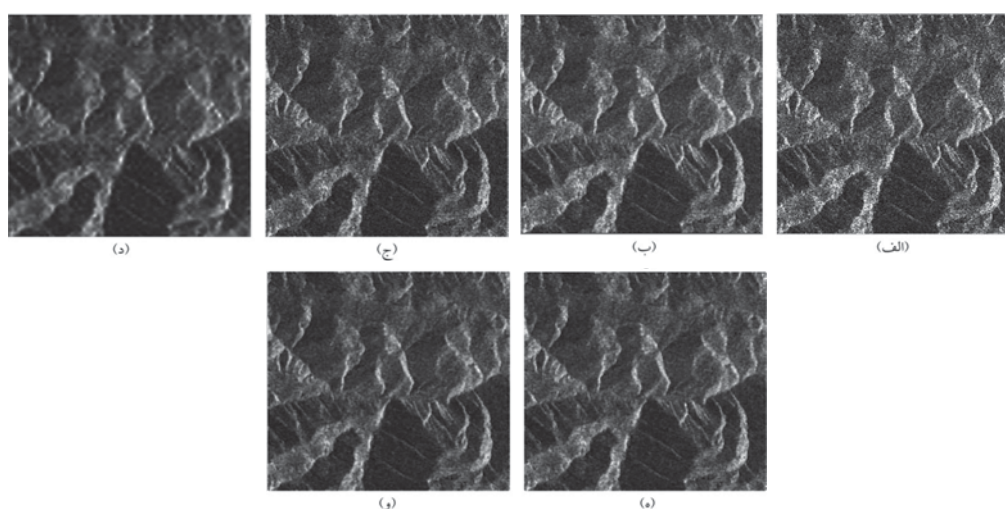
شکل ۳- مقایسه روش‌های حذف نوفه اسپیکل بر روی یک تصویر واقعی (الف: SAR: تصویر نوفه‌ای، (ب) روش لی، (ج) روش وینر، (د) روش آستانه‌گذاری نرم ضرایب موجک، (ه) روش WINSAR، (و) روش پیشنهادی
