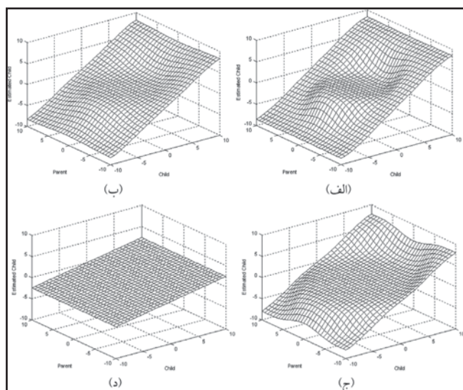
شکل ۱- رویه ورودی- خروجی پردازنده بیز پیشنهادی در رابطه (۱۵) به ازای نسبت ثابت \sigma_{\eta}^2/\gamma=2.5 و چهار مقدار مختلف \alpha : الف) \alpha=0.5 ، ب) \alpha=1.5 ، ج) \alpha=1.95 و د) \alpha=2 .
