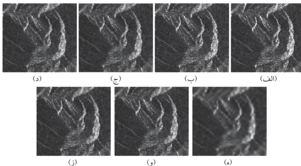
شکل ۲- مقایسه نتایج حذف نوفه اسپیکل شبیه‌سازی شده توسط روش‌های مختلف: (الف) تصویر بدون نوفه (ب) تصویر نوفه‌ای با نسبت سیگنال به نوفه ۱۰/۴۶ دی بی، (ج) روش لی، (د) روش وینر، (ه) روش آستانه‌گذاری نرم ضرایب موجک، (و) روش WINSAR، (ز) روش پیشنهادی
