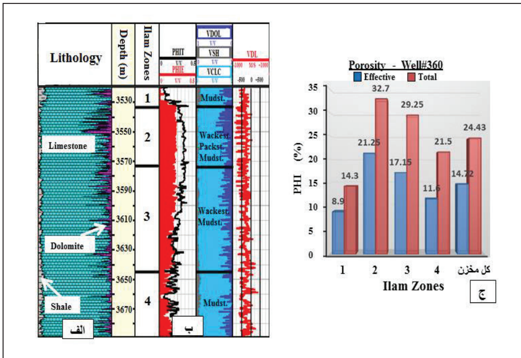
شکل ۱۱- الف و ب) مقایسه تغییرات پارامترهای پتروفیزیکی در زون‌های مختلف: تخلخل کل، تخلخل مؤثر، حجم شیل، رس و دولومیت همراه با نمودار انحراف سرعت در ستون چینه‌ای مربوطه؛ ج) تغییرات ستونی تخلخل مؤثر و کل.
