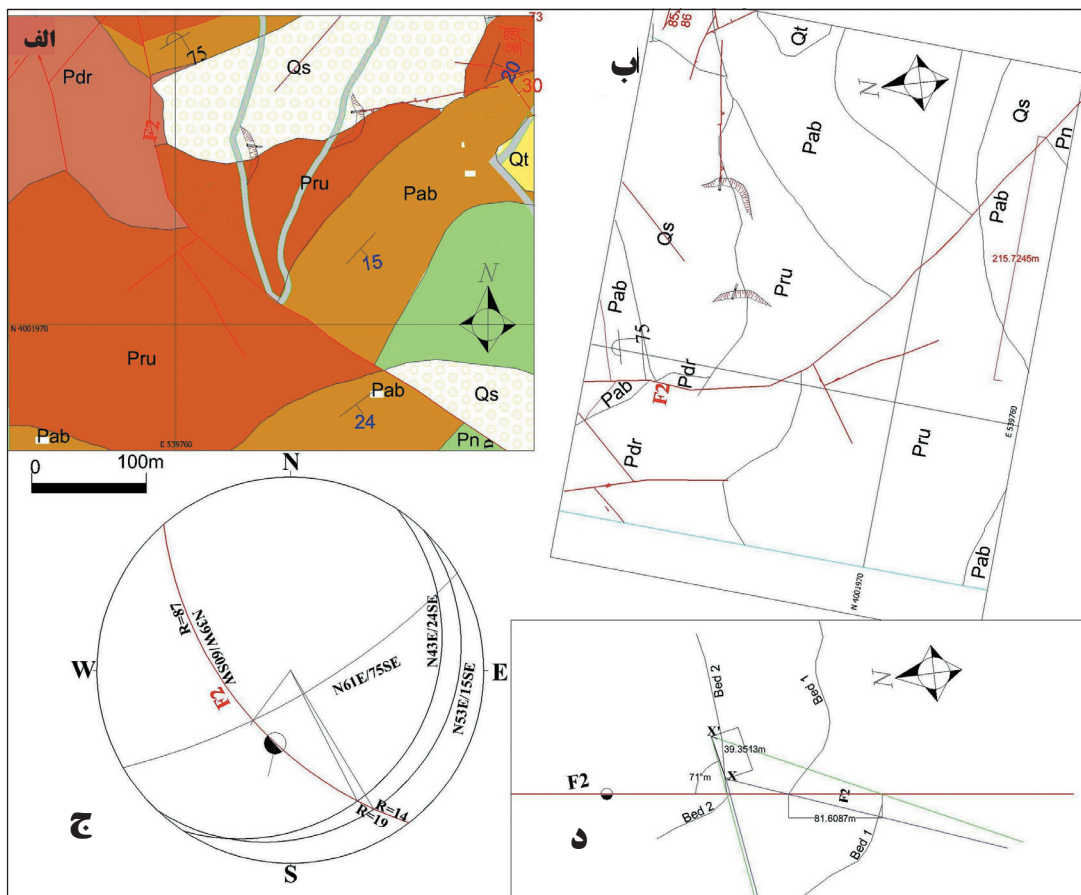
شکل ۹- تحلیل فضایی گسل F2 با استفاده از نقشه زمین شناسی شکل ۴ و شبکه اشمیت و روش ترسیم (روش مطالعه اقباس شده از Ragan, 1973).
