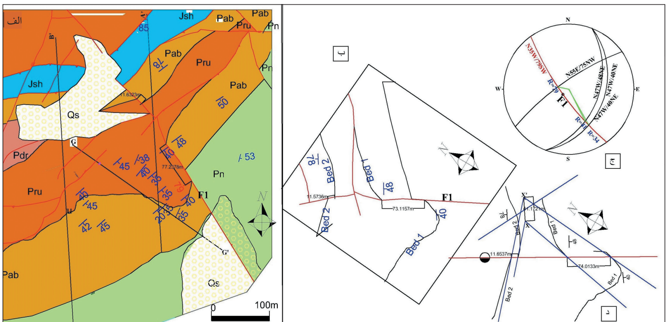
شکل ۸- تحلیل فضایی گسل F1 با استفاده از نقشه زمین‌شناسی شکل ۴ و شبکه اشمیت و روش ترسیمی (روش مطالعه اقتباس شده از Ragan, 1973).
