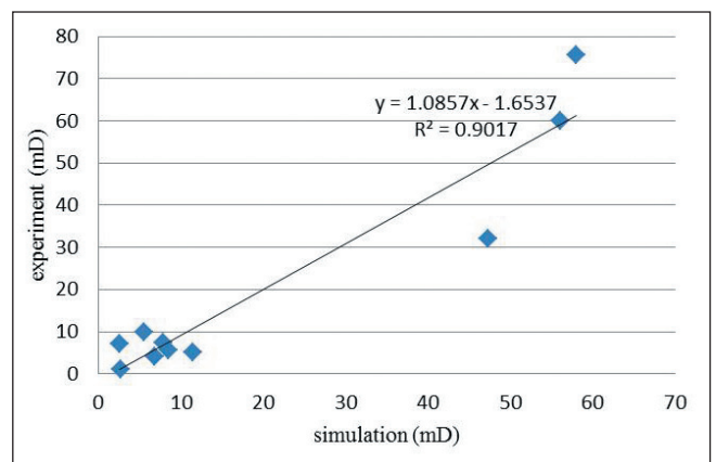
شکل ۱۱- نمودار تراوایی اندازه‌گیری شده بر حسب تراوایی تخمین زده شده.
