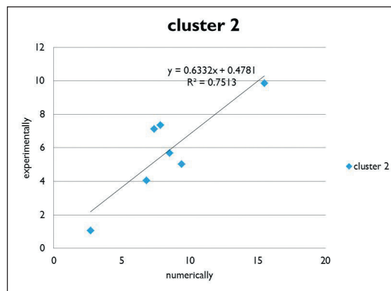
شکل ۱۳- نمودار تراوایی اندازه‌گیری شده بر حسب تراوایی تخمین زده شده برای تراوایی کمتر از ۳۰ میلی داری.
