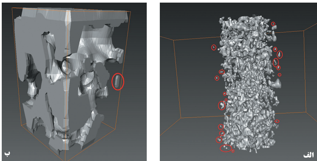
شکل ۵- اتصال فضاهای خالی؛ الف) در مقیاس ۲۰۰ در ۲۰۰ در ۹۷ و کسل؛ ب) در مقیاس ۴۰ در ۴۰ در ۲۰ و کسل.
