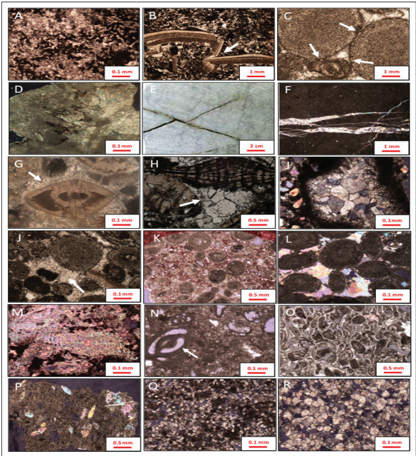
شکل ۳- تصاویر میکروسکوپی فرایندهای دیاژنزی در رخساره‌های کربناته. (A) به دام افتادن میکربت در حجرات باندستون مرجانی، آغاچاری ۶۴، عمق ۲۳۹۹ متری. نمونه توسط آلزارین قرمز رنگ آمیزی شده است؛ (B) شکستگی صدف دوکفه‌ای تحت تأثیر فشردگی فیزیکی، آغاچاری ۳۰، عمق ۲۰۸۵ متری؛ (C) ایجاد حاشیه میکربیتی در اطراف آئیدها در نتیجه فرایند میکربیتی شدن و تماس نقطه‌ای آنها با یکدیگر تحت تأثیر فشردگی فیزیکی، آغاچاری ۳۰، عمق ۲۰۳۷ متری؛ (D) تجمع مواد آلی و کانی‌های رسی در امتداد استیلولیت دامنه کوتاه در نتیجه فشردگی شیمیایی، آغاچاری ۶۶، عمق ۲۸۱۰ متری؛ (E) شکستگی‌های مزدوج باز در مغزه‌های حفاری، آغاچاری ۳۰، عمق ۱۹۷۳ متری؛ (F) شکستگی‌های پرشده توسط سیمان انیدریتی، آغاچاری ۶۱، عمق ۲۵۵۲ متری؛ (G) سیمان حاشیه‌ای هم‌ضخامت بر روی دیواره خارجی فسیل روتالیا (فلش)، چاه ۳۰، عمق ۲۰۹۷ متری؛ (H) تشکیل سیمان حاشیه‌ای هم‌ضخامت بر روی دیواره فسیل‌ها و ادامه یافتن آن توسط سیمان هم‌بعد، آغاچاری ۳۰، عمق ۲۲۶۲ متری؛ (I) باقی ماندن حاشیه میکربیتی فسیل انحلال یافته و پر شدن آن توسط سیمان کلسیت دروزی، آغاچاری ۳۰، عمق ۲۱۴۸ متری؛ (J) سیمان هم‌بعد پرکننده فضاهای خالی بین آئیدها (فلش)، آغاچاری ۳۰، عمق ۲۰۲۰ متری؛ (K) سیمان پوریکلو تاپیک در برگیرنده دانه‌های آئید. نمونه توسط آلزارین قرمز رنگ آمیزی شده است. آغاچاری ۳۰، عمق ۲۰۳۷ متری؛ (L) سیمان انیدریتی بین دانه‌ای در فضای بین آئیدها، آغاچاری ۳۰، عمق ۲۰۲۰ متری؛ (M) حفظ شدگی کامل ساختار فسیل‌های لیدوسیکلینا و میلیولید در اثر فرایند انیدریتی شدن، آغاچاری ۱۴۹، عمق ۲۸۲۰ متری؛ (N) حفظ شدن حاشیه میکربیتی و ایجاد تخلخل قالبی در فسیل میلیولیده در نتیجه فرایند انحلال. آغاچاری ۶۶، عمق ۲۶۷۴ متری؛ (O) انحلال غیر انتخابی فسیل‌ها و سیمان، آغاچاری ۶۱، عمق ۲۶۶۵ متری؛ (P) دولومیت‌های خیلی ریزبلور دارای فابریک فنسترال و قالب‌های تبخیری، آغاچاری ۶۶، عمق ۲۷۱۰ متری؛ (Q) فضاهای بین بلورین در دولومیکرواسپارها، آغاچاری ۱۴۹، عمق ۲۶۶۵ متری؛ (R) بلورهای درشت دولومیت با مراکز ابری و حاشیه‌های شفاف، آغاچاری ۶۱، عمق ۲۵۵۳ متری. تصاویر میکروسکوپی G، H و K و PPL و بقیه در XPL تهیه شده است.
