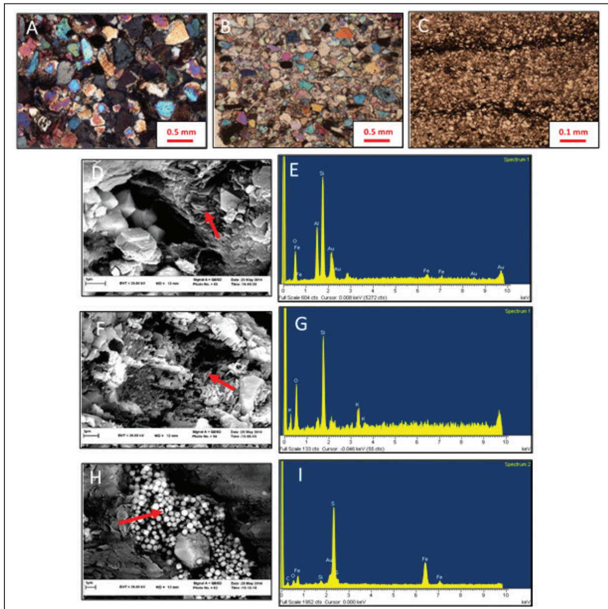
شکل ۴- تصاویر میکروسکوپی فرایندهای دیاژنزی در رخساره‌های آواری. (A) تماس محدب-مقعر دانه‌های کوارتز تحت تأثیر فشردگی فیزیکی، پتروفاسیس E، آغاچاری ۱۴۹، عمق ۲۷۳۹ متری؛ (B) سیمان کلسیتی فراگیرنده دربرگیرنده دانه‌های کوارتز، آغاچاری ۱۴۹، عمق ۲۷۱۴ متری؛ (C) سیمان اکسید آهن در رخساره کوارتز آرنایت، آغاچاری ۱۴۹، عمق ۲۷۴۸ متری؛ (D و E) تصویر میکروسکوپ الکترونی همراه با آنالیز نقطه‌ای (محل فلش) از کانی رسی کائولینیت با بافت کتابی در رخساره ماسه سنگ میکربیتی، آغاچاری ۳۰، عمق ۲۲۹۰ متری؛ (F و G) وجود کانی رسی ایلیت با حالت پرمزمانند همراه با آنالیز نقطه‌ای (محل فلش) که باعث پرشدن فضاهای خالی در رخساره ماسه سنگ میکربیتی شده است. آغاچاری ۶۶، عمق ۲۷۱۶ متری؛ (H و I) تصویر میکروسکوپ الکترونی از پیریت‌های دانه تمشکی همراه با آنالیز نقطه‌ای (محل فلش) در رخساره کوارتز آرنایت، آغاچاری ۱۴۹، عمق ۲۷۵۶ متری. تصاویر میکروسکوپی A و B در XPL و تصویر C در PPL تهیه شده است.
