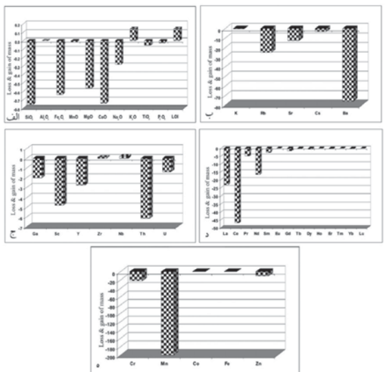
شکل ۴- هیستوگرام‌های تغییرات جرم در زون دگرسانی پروپلیتی؛ الف) اکسیدهای اصلی، ب) LHFSE، ج) HFSE، د) REEها، ه) FTSMها
