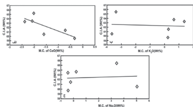
شکل ۱۰- نمودارهای دومتغیره تغییر جرم الف) CaO، ب) K 2 O و ج) Na 2 O در برابر CIA (شاخص شیمیایی دگرسانی) در توده گرانیتوبیدی آستانه
