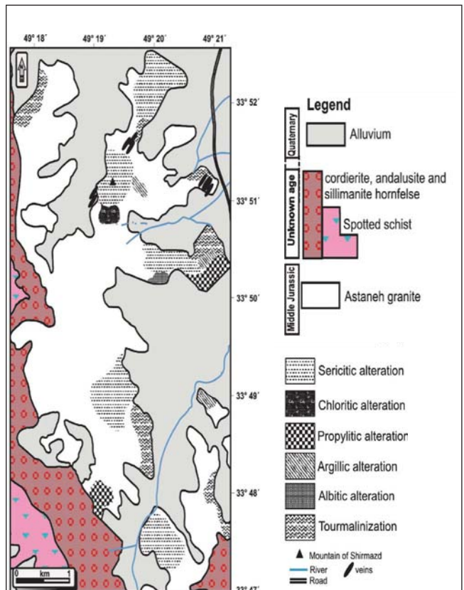
شکل ۲- نقشه دگرسانی توده گرانیتیویدی آستانه
