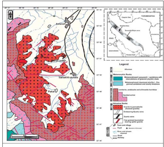
شکل ۱- نقشه زمین شناسی توده گرانیتیویدی آستانه (سهنی و همکاران، ۱۳۸۵)
