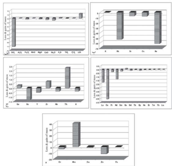
شکل ۵- هیستوگرام‌های تغییرات جرم در زون دگرسانی آرژیلیتی؛ الف) اکسیدهای اصلی، ب) LHFSE، ج) HFSE، د) REEها، ه) FTSMها
