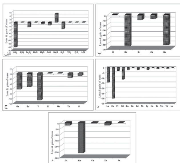
شکل ۷- هیستوگرام‌های تغییرات جرم در زون دگرسانی آلبیتی؛ الف) اکسیدهای اصلی، ب) LFSEها، ج) HFSEها، د) REEها، ه) FTSMها
