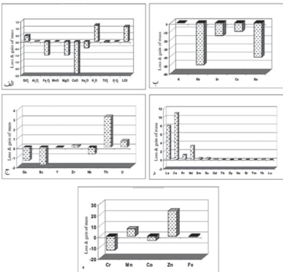
شکل ۳- هیستوگرام‌های تغییرات جرم در زون دگرسانی سریستی؛ الف) اکسیدهای اصلی، ب) LHFSE، ج) HFSE، د) REEها، ه) FTSMها
