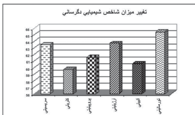
شکل ۹- تغییر میزان شاخص شیمیایی دگرسانی در زون‌های دگرسانی منطقه آستانه
