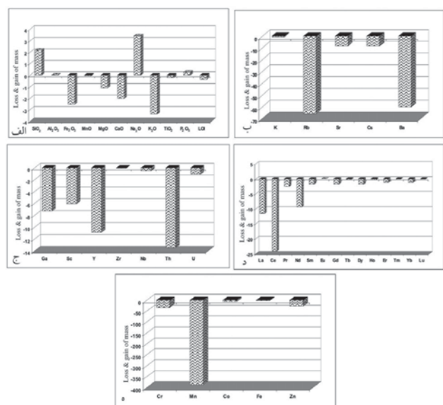
شکل ۸- هیستوگرام‌های تغییرات جرم در زون دگرسانی تورمالینی؛ الف) اکسیدهای اصلی، ب) LFSEها، ج) HFSEها، د) REEها، ه) FTSMها
