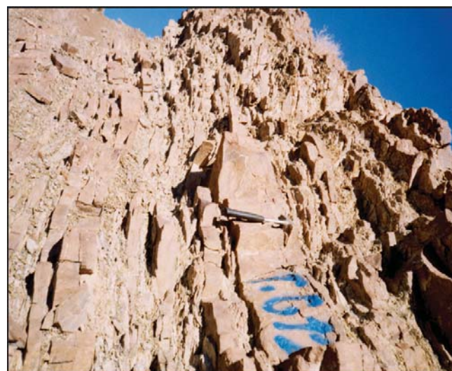
شکل ۸- ماسه سنگ‌های قهوه‌ای رنگ دارای آثار رپیل مارک و ایکنوفسیل‌های cruziana isp. در تناوب با شیل‌های سبز رنگ بخش بالایی عضو شیل زیرین سازند شیرگشت در برش میوگدار - جهت دید به سمت خاور
