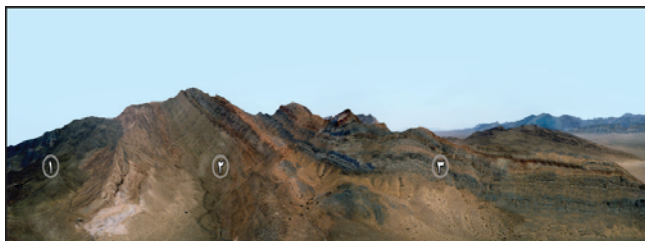
شکل ۵- نمای کلی از سازندهای کلمرد (۱)، شیرگشت (۲) و گچال (۳) در بلندی‌های کلمرد و محل برش میوگدار - جهت دید به سمت شمال خاوری
