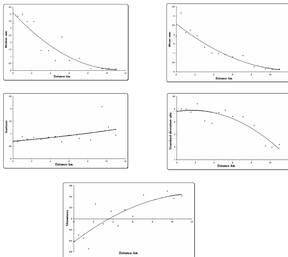
شکل ۴- نمودار تغییرات طولی پارامترهای الف) میانگین، ب) میانه، ج) جورشدگی، د) کج شدگی و ه) کشیدگی اندازه ذرات در نمونه های برداشت شده از رودخانه لاثشور
