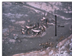
شکل ۵- ساختمانهای رسوبی مشاهده شده در حوضه آبخیز لاثشور، الف) طبقات توده ای، ب) موج نقش نامتقارن، ج) طبقه بندی تدریجی با بافت برگشتی، د) ترکهای گلی و ه) ساختمانهای کنده شده و پر شده
