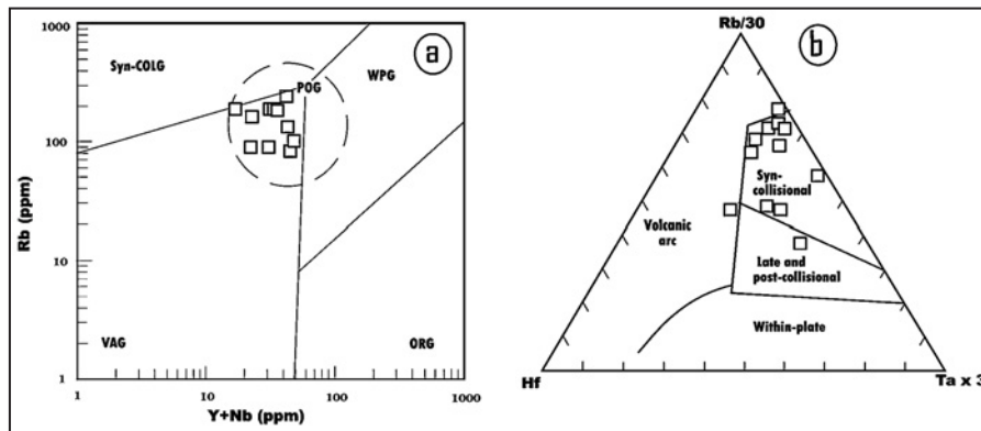
شکل ۷- (a) موقعیت نمونه‌های توده سیه‌کمر در نمودار Y+Nb در برابر Rb (Pearce, 1996) و (b) نمودار Rb/30-Hf-Ta (Harris et al., 1986) برای رده‌بندی گرانیتوئیدها (VAG=گرانیت‌های کمان آتشفشانی؛ Syn-COLG=گرانیت‌های همزمان با برخورد و POG=گرانیت‌های پس از برخورد).
