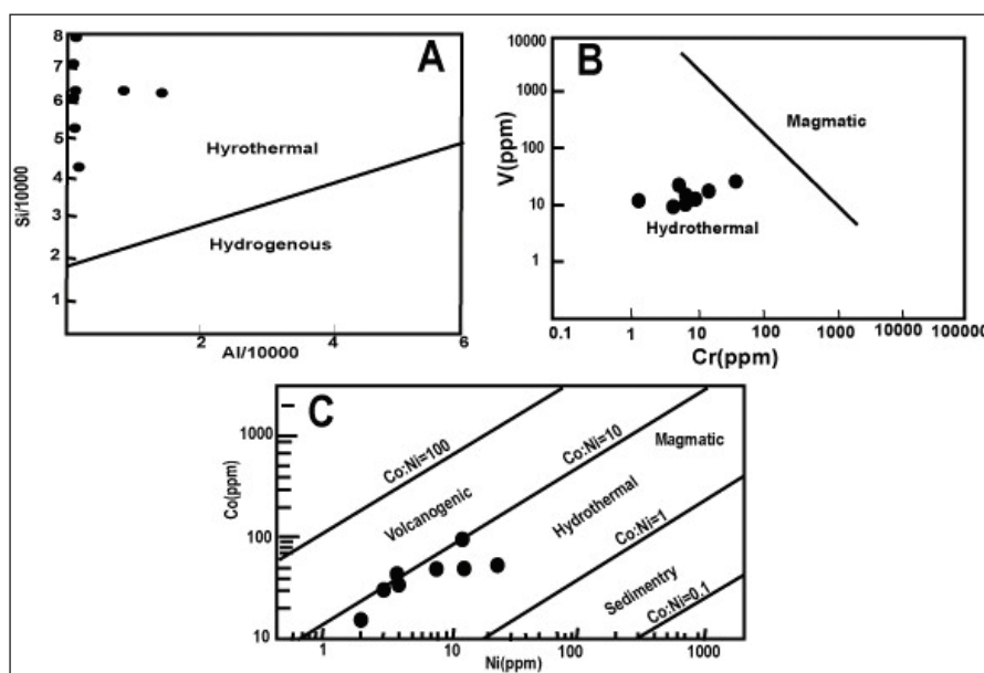
شکل ۱۱- A) نمودار نسبت Co در برابر Ni و چگونگی قرارگیری نمونه‌های کانسنگ منیتیت و تعیین منشأ کانسار که نشان‌دهنده نوع کانی‌سازی منیتیت در سیستم گرمایی می‌باشد (Bajwa et al., 1987). B) نسبت V در برابر Cr که نشان‌دهنده قرارگیری و شکل‌گیری نوع کانی‌سازی گرمایی است. C) تغییرات نسبت Al به Si و قرارگیری بیشتر نمونه‌ها در محدوده کانسار آهن با منشأ گرمایی است (با توجه به تعداد بیشتر نمونه‌هایی که فقط از آنالیز شیمی تر برخوردار بوده اند از این نمودار استفاده شده است) (Beaudoin and Dupuis, 2011).
