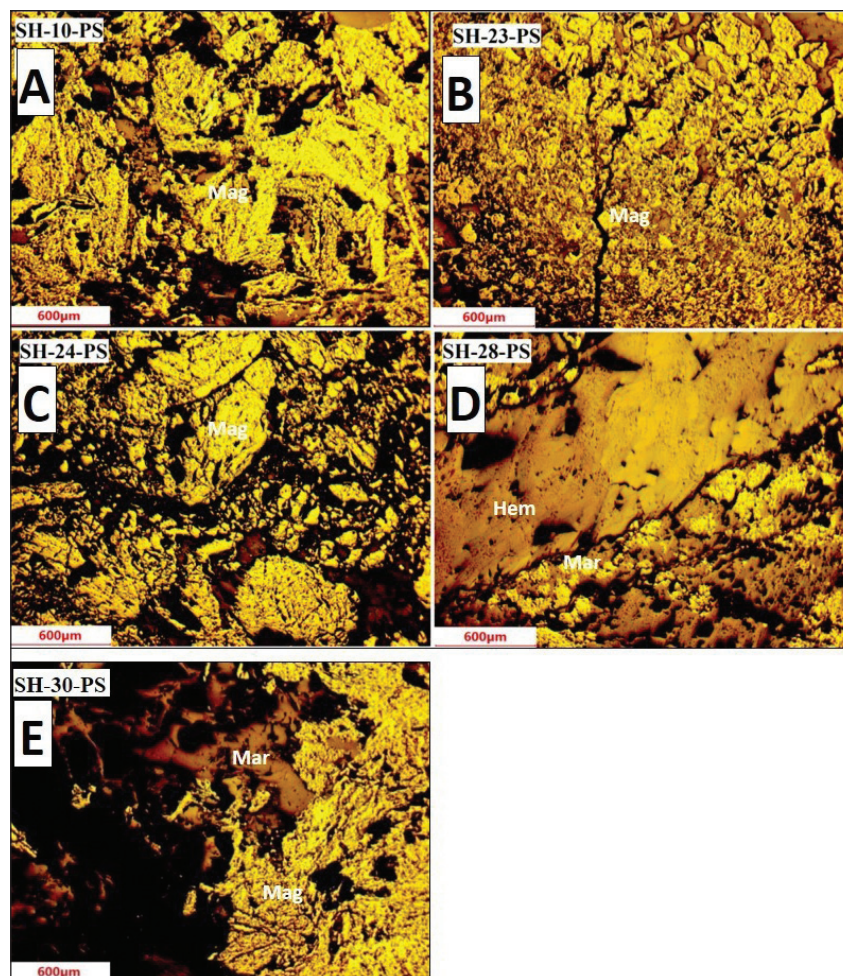
شکل ۵- A) کانه منیتیت (Mag) با تجمعات شعاعی و سوزنی شکل که در بعضی بخش ها تبدیل به هماتیت (Mar) شده است. B) ذرات کانی های ریز، عموماً خود شکل منیتیت (Mag) همراه با فرایند مارتیتی شدن (Mar) بسیار ضعیف. C) نمونه از ۸۰٪ حجمی منیتیت (Mag) تشکیل شده است. D) مارتیتی شدن منیتیت و همچنین رگه هماتیت (Hem) که کانه منیتیت (Mag) را به صورت ثانویه قطع کرده است. E) منیتیت که در حاشیه به هماتیت تبدیل شده است (Whitney and Evans, 2010).
