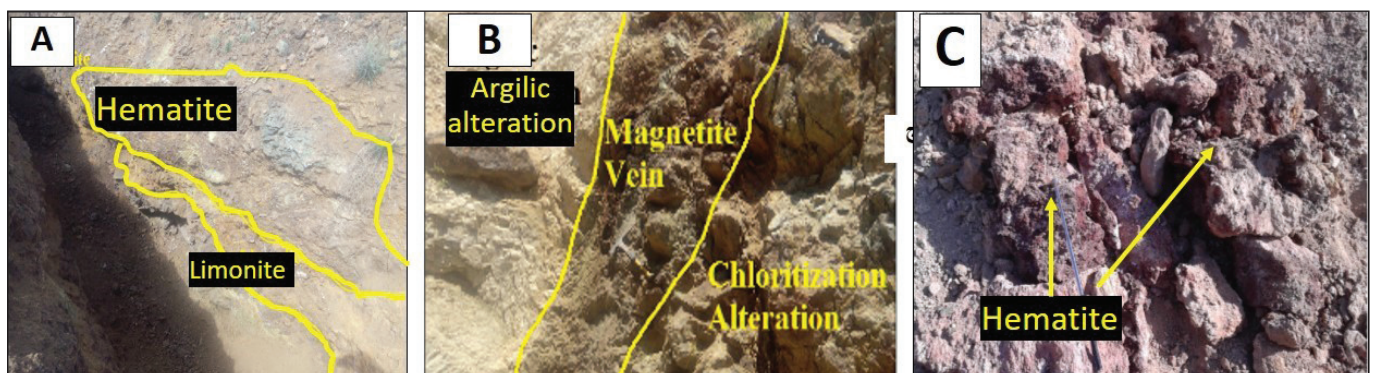
شکل ۵- (A) ترانشه حفر شده در محدوده مورد مطالعه در زون اکسید آهنی و آثار هماتیت و لیمونیت در آن (دید به سمت شمال خاور). (B) دگرسانی کلریتی و آرژیلیک و کانی زایی اکسید آهن در کنتاکت بین واحدهای کربناتی و شیستی در بخش جنوبی محدوده یاپل (دید به سمت شمال خاور). (C) دگرسانی هماتی و گسترش آن (دید به سمت شمال).
