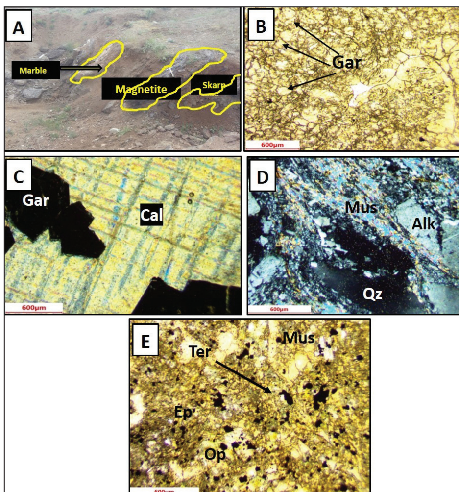
شکل ۳- (A) سنگ‌های اسکارنی و کانی‌سازی آهن به شکل عدسی شکل در درون آنها (دید به سمت شمال باختر). (B) اسکارن با بافت گرانو بلاستیک تا پورفیرو بلاستیک و کانی‌های گارنت (Gar) همراه با کلسیت با کانی‌های فرعی اپیک وجود دارد. (C) کانی کلسیت (Cal) همراه با کانی گارنت (Gar) به صورت درشت دانه. (D) گنیس یا میلونیت معادل رخساره دگرگونی شیب سبز با بافت گرانوبلاستیک - سایه فشاری (Pressure shadow) (چشمی یا اوگن Qz) همراه با پلاژیوکلاز به مقدار کم و آلکالی فلدسپار (Alk) به صورت درشت بلور دیده می‌شود. (E) متاسوماتیت با بافت گرانولار و کانی‌های مسکوویت (Mus)، مقادیر اندکی ترمولیت (Ter) اکتینولیت و اپیدوت (Ep) و کانی‌های اپیک (Op) در مقطع دیده می‌شود (Whitney and Evans, 2010).
