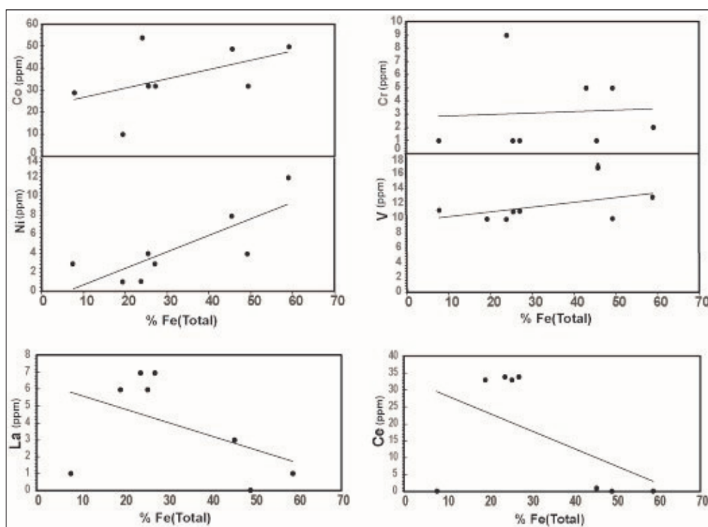
شکل ۱۰- تغییرات مقدار عناصر کبالت، کروم، نیکل، وانادیم با شیب تغییرات مثبت و لانتانیم، سربیم را با شیب تغییرات منفی نسبت به درصد آهن نشان می دهد.
