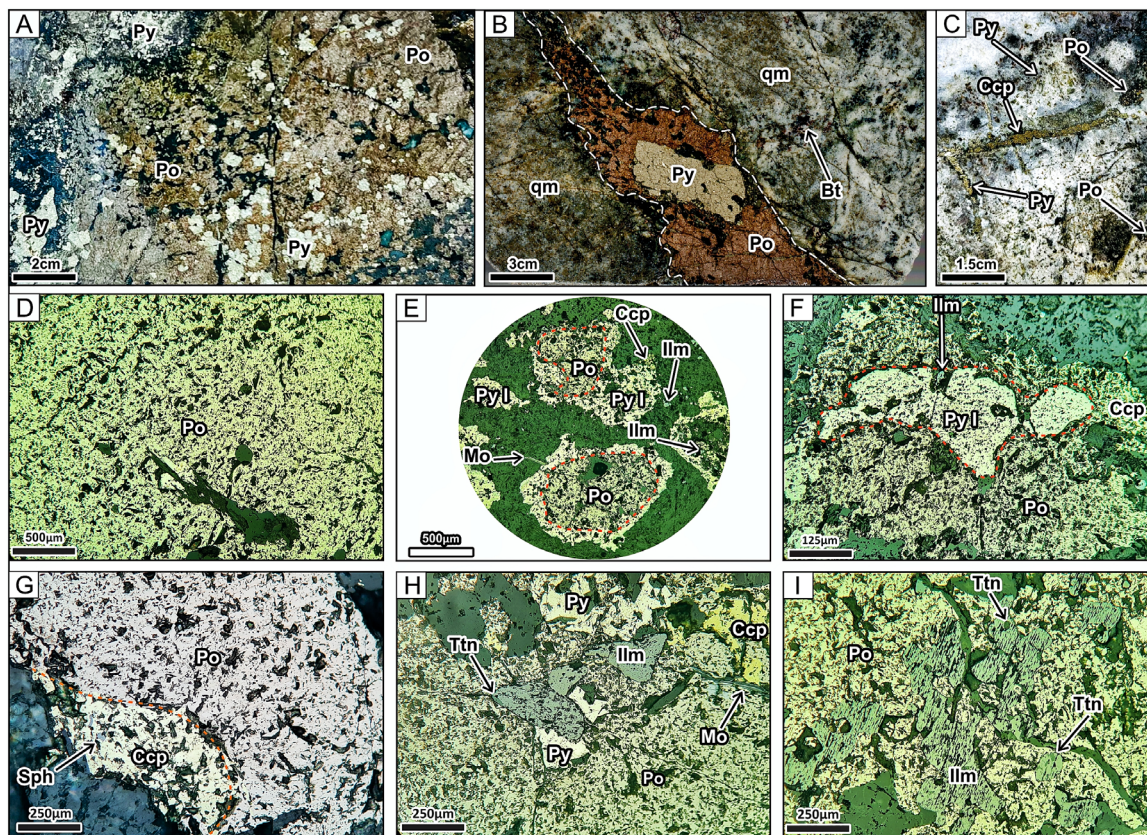
شکل ۱۳- تصاویر نمونه دستی و میکروسکوپی از رخداد کانی‌های فلزی در دگرسانی پتاسیک، (A) تصویر نمونه دستی از کانی‌های سولفیدی پیروتیت (Po) و پیریت (Py) با بافت توده‌ای؛ (B) نمونه دستی از رخداد رگچه‌های پیروتیت (Po) و پیریت (Py) در همراهی با توده کوآرتز مونزونیتی؛ (C) نمونه دستی از رخداد رگچه‌های کالکوپیریت (Ccp)، پیروتیت (Po) و پیریت (Py) در همراهی با دگرسانی پتاسیک؛ (D) تصویر میکروسکوپی از رخداد پیروتیت (Po) با بافت توده‌ای؛ (E) تصویر میکروسکوپی از کانی پیروتیت (Po) که از اطراف و به‌طور بخشی توسط پیریت فاز اول (Py)، کالکوپیریت (Ccp) و مولیبدنیت فاز اول (Mo I) جانشین شده است. ایلمنیت (Ilm) با بافت دانه‌پراکنده، کانی‌های سولفیدی را همراهی می‌کند؛ (F) تصویر میکروسکوپی از پیریت فاز اول (Py I) که پیروتیت (Po) جانشین آن شده است. در اطراف، کانی کالکوپیریت (Ccp) نیز تشکیل شده است؛ (G) تصویر میکروسکوپی از کانه‌زایی با بافت توده‌ای از پیروتیت (Po)، کالکوپیریت (Ccp) و اسفالریت (Sph) که هم‌رشدی نشان می‌دهند. (H) تصویر میکروسکوپی از رخداد کانی‌های ایلمنیت (Ilm)، تیتانیت (Ttn)، کالکوپیریت (Ccp) و پیریت (Py) با بافت توده‌ای و به‌صورت هم‌رشد تشکیل شده‌اند؛ (I) تصویر میکروسکوپی از رخداد کانی‌های ایلمنیت (Ilm) و پیروتیت (Po) هم‌رشدی نشان می‌دهند و کانی ایلمنیت در حال جانشین شدن توسط تیتانیت (Ttn) است.
