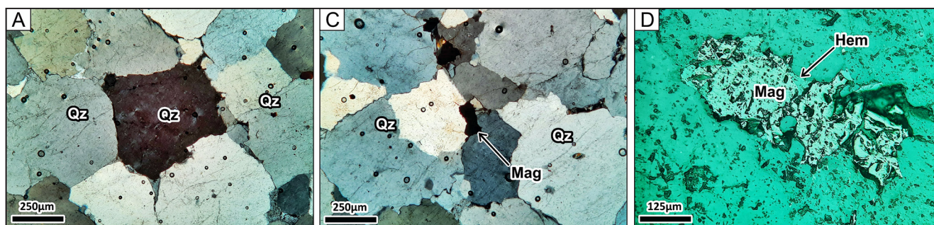
شکل ۶- تصاویر میکروسکوپی از دگرسانی سیلیسی (نورهای عبوری و انعکاسی با نیکول‌های متقاطع (XPL)، A و B) تصاویر میکروسکوپی از دگرسانی سیلیسی، که از بلورهای درشت تا متوسط کوارتز (Qz) تشکیل شده است؛ C) رخداد کانی‌های مگنتیت (Mag) و هماتیت (Hem) که همزمان با دگرسانی سیلیسی تشکیل شده‌اند.
