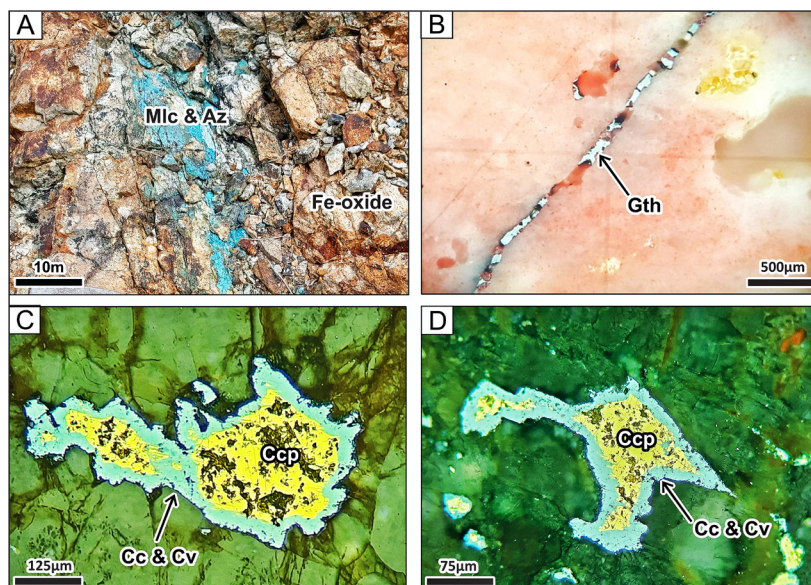
شکل ۱۸- A) تصویر رخنمون از کانی‌سازی مس اکسیدی با رخداد مالاکیت (Mlc) و آزوریت (Az) همراه با ترکیبات هیدروکسیدی آهن (Fe-oxide) در توده کوارتز مونزونیتی دگرسان شده؛ B) تصویر میکروسکوپی از گوتیت، که به صورت رگچه و نیز جانشینی پیریت‌های اکسایش یافته مشاهده می‌شود؛ C و D) تصاویر میکروسکوپی از رخداد کانی‌های کالکوپریت (Ccp)، که از حاشیه بلورها و مرز شکستگی‌ها توسط کالکوسیت (Ccs) و کوولیت (Cv) جانشین شده‌اند.
