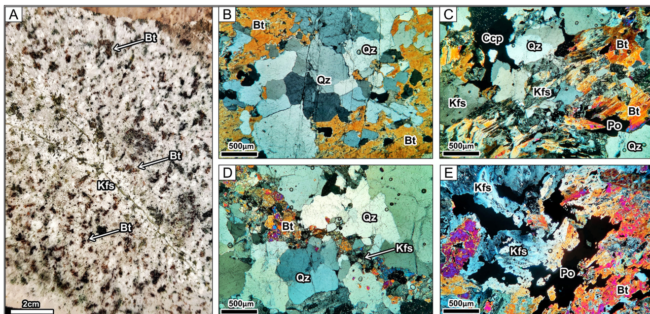
شکل ۷- تصاویر نمونه دستی و میکروسکوپی از دگرسانی پتاسیک؛ A) تصاویر نمونه دستی از توده کوارتز مونزونیتی تا کوارتز مونزودیوریتی که متحمل دگرسانی پتاسیک شده است و حاوی کانی‌های بیوتیت (Bt) و آلکالی‌فلدسپار (Kfs) است؛ B و C) تصاویر میکروسکوپی از دگرسانی‌های سیلیسی مرحله اول و پتاسیک، که کانی‌های بیوتیت (Bt)، آلکالی‌فلدسپار (Kfs)، کالکوپریت (Ccp) و پیرویت (Po) دگرسانی پتاسیک در بین بلورهای کوارتز (Qz) دگرسانی سیلیسی مرحله اول جایگیر شده‌اند؛ D) رگچه حاوی کانی‌های بیوتیت (Bt) و آلکالی‌فلدسپار (Kfs) که کانی‌های کوارتز (Qz) دگرسانی سیلیسی مرحله اول را قطع کرده است؛ E) تصاویر میکروسکوپی از آلکالی‌فلدسپار (Kfs) و بیوتیت‌های (Bt) دگرسانی پتاسیک.
