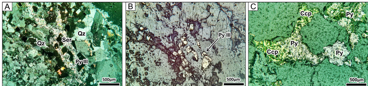
شکل ۱۷- A و B) رخداد بلورهای کوارتز (Qz) و سریسیت (Ser) گویای دگرسانی فلیک که دارای کانی‌سازی سولفیدی پیریت (Py) است؛ C) تصویر میکروسکوپی از پهنه دگرسانی فلیک با بلورهای پیریت (Py) و کالکوپریت (Ccp).
