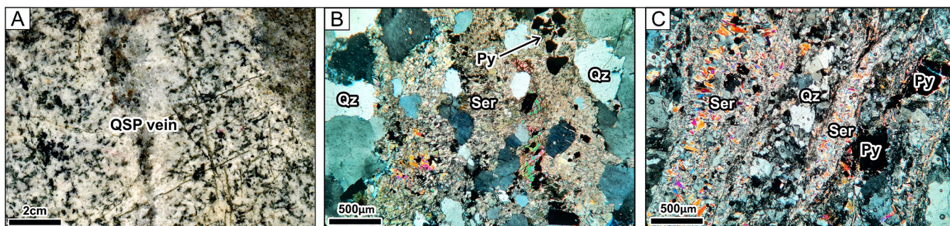
شکل ۸- تصاویر میکروسکوپی از دگرسانی فیلیک. (A) رگچه مرتبط با دگرسانی فیلیک در توده تونالیتی در مقیاس نمونه دستی که تشکیل فراگیر کوارتز با بافت رگچه‌ای و دانه‌پراکنده را نشان می‌دهد؛ (B و C) تصاویر نور عبوری از رخدادهای کانی‌های سریست (Ser) و کوارتز (Qz) در همراهی با پیریت (Py).
