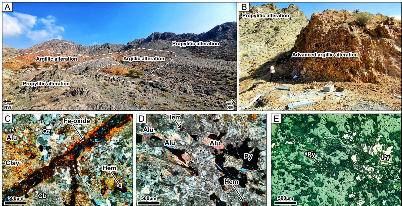
شکل ۹- تصاویر صحرایی و میکروسکوپی از رخداد دگرسانی آرژلیک؛ (A) تصویر دورنما از رخنمون دگرسانی آرژلیک که توسط دگرسانی پروپلیتیک احاطه شده است؛ (B) نمای از گسترش دگرسانی‌های آرژلیک پیشرفته و پروپلیتیک؛ (C) تصویر میکروسکوپی از رخداد کوارتز (Qz)، کانی‌های رسی (Clay)، کربنات (Cb) و رگچه اکسید آهن (Fe-Oxide) در طی دگرسانی آرژلیک؛ (D) تصویر میکروسکوپی از رخداد دگرسانی آرژلیک پیشرفته که با تشکیل کانی‌های رسی (Clay)، کربنات (Cb) و آلونیت (Alu) همراه است؛ (E) همان تصویر "D" در نور انعکاسی، که رخداد پیریت (Py) و هماتیت (Hem) در زمینه‌ای از کانی آلونیت (Alu) را نشان می‌دهد.
