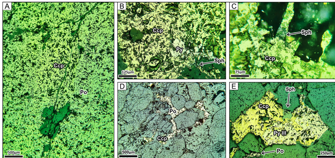
شکل ۱۴- تصاویر میکروسکوپی در نور انعکاسی از رخداد کالکوپیریت در پهنه دگرسانی پتاسیک. (A) هم‌رشدی کالکوپیریت (Ccp) و پیروتیت (Po) با بافت توده‌ای؛ (B) هم‌رشدی پیریت (Py) و کالکوپیریت (Ccp) با بافت توده‌ای که حاوی ادخال‌هایی از اسفالریت (Sph) است؛ (C) تصاویری از روابط بافتی کالکوپیریت (Ccp) و ادخال‌های کوچک اسفالریت (Sph)؛ (D) کانی‌های کالکوپیریت (Ccp) و پیروتیت (Po) با بافت رگچه‌ای؛ (E) هم‌رشدی کالکوپیریت (Ccp)، پیروتیت (Po)، پیریت فاز سوم (Py III) و اسفالریت (Sph) که در مرز بلورهای کوارتز سیلیسی شدن مرحله اول تزریق شده‌اند.
