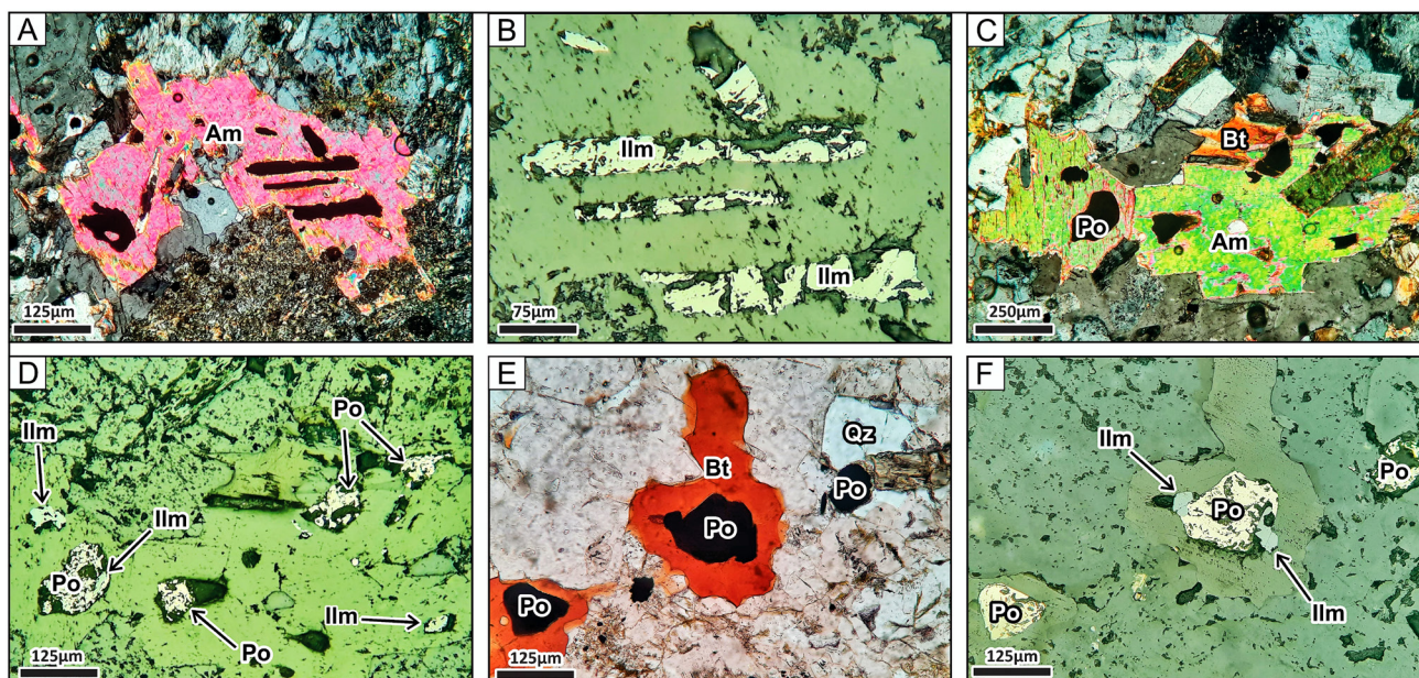
شکل ۱۲- تصاویر میکروسکوپی از کانی‌های همراه در توده نفوذی کوآرتز مونزونیتی - کوآرتز مونزودیوریتی. A و B) به ترتیب تصاویر میکروسکوپی نور عبوری و نور انعکاسی از کانی آمفیبول (Am) که ایلمنیت (Ilm) به صورت ادخال در داخل آمفیبول ژرف‌زاد تشکیل شده است؛ C و D) تصاویر میکروسکوپی از رخداد ایلمنیت (Ilm) و پیرویت (Po) به صورت ادخال در آمفیبول؛ E و F) به ترتیب تصاویر میکروسکوپی نور عبوری و نور انعکاسی از هم‌رشدی ایلمنیت (Ilm) و پیرویت (Po) در داخل بلورهای بیوتیت (Bt) و کوآرتز (Qz).
