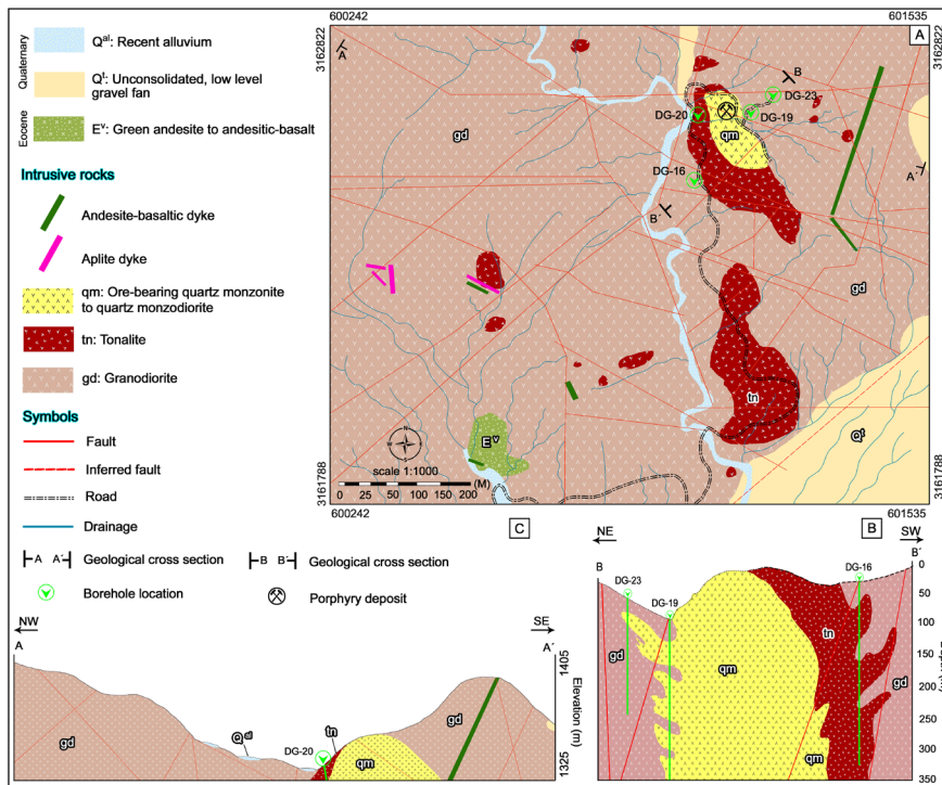
شکل ۳- A) نقشه زمین‌شناسی- ساختاری کانسار مس دهنه‌گمرکان با مقیاس ۱:۱۰۰۰؛ B و C) مقاطع زمین‌شناسی B-B' و A-A'، که نحوه ارتباط توده‌های نفوذی با یکدیگر را نشان می‌دهد (با تغییرات افشون و همکاران، ۱۴۰۲).
