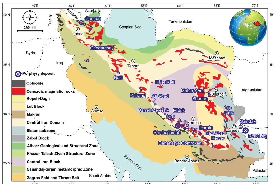
شکل ۱- نقشه زمین‌شناسی- ساختاری ایران که توزیع ذخایر مس پورفیری را با نمادهای دایره‌ای شکل نشان می‌دهد (نقشه زمین‌شناسی و ساختاری ایران با اصلاحات از آغانباتی (Aghanabati, 1998, 2004)، علوی (Alavi, 1996)، ریچاردز و شعله (Richards and Sholeh, 2016)).
