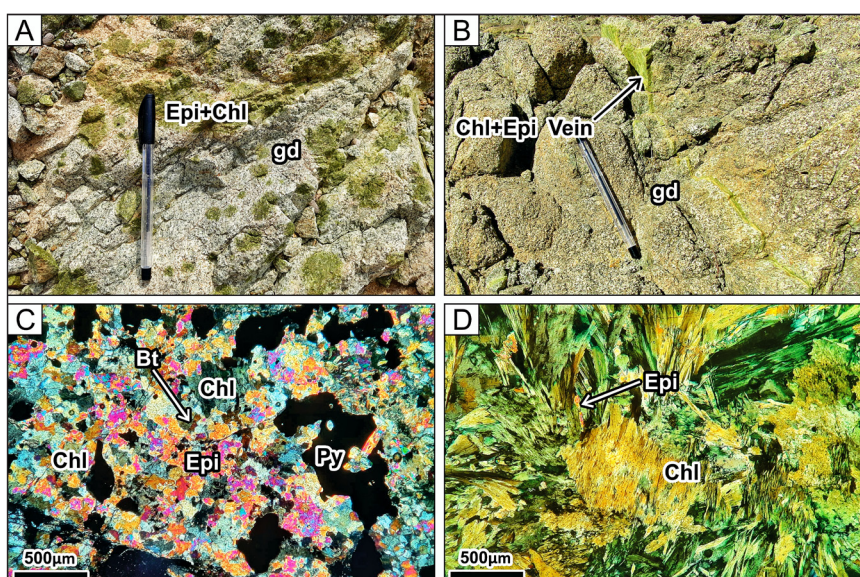
شکل ۱۰- تصاویر نمونه دستی و میکروسکوپی از رخداد دگرسانی پروپلیتیک؛ (A) نمای نزدیک از رخداد دگرسانی پروپلیتیک در توده گرانودیوریتی که با کانی‌های کلریت (Chl) و اپیدوت (Epi) همراه است؛ (B) نمای از رگه اپیدوتی (Epi) و کلریتی (Chl) که توده گرانودیوریتی را قطع کرده است؛ (C) تصویر میکروسکوپی از همراهی کانی‌های کلریت (Chl)، اپیدوت (Epi)، بیوتیت (Bt) و پیریت (Py) در نمونه دگرسان شده پروپلیتیک؛ (D) تصویر میکروسکوپی دیگر از رخداد قابل توجه بلورهای سبز رنگ کلریت (Chl) همراه با مقادیر جزئی اپیدوت (Epi).
