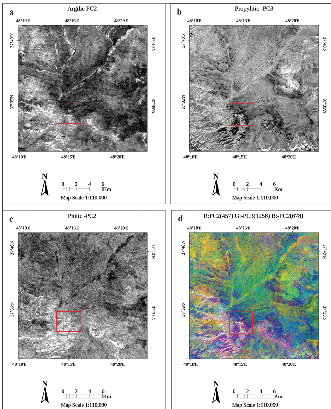
شکل ۶- پردازش تصاویر سنجنده استر به روش کروستا: (a) تصویر (PC2) مربوط به ترکیب باندهای ۴، ۵، ۷؛ پیکسل‌های روشن در تصویر نشان‌دهنده دگرسانی آرژیلیک در منطقه می‌باشند. (b) تصویر (-PC3) مربوط به ترکیب باندهای ۱، ۲، ۵، ۸؛ پیکسل‌های روشن نشان‌دهنده دگرسانی پروپیلیتی در منطقه می‌باشند. (c) تصویر (-PC2) مربوط به ترکیب باندهای ۶، ۷، ۸؛ پیکسل‌های روشن نشان‌دهنده دگرسانی فلیک در منطقه می‌باشند. (d) ترکیب رنگی کاذب (R: PC2(457), G: -PC3(1258), B: -PC2(678)) که در منطقه مورد مطالعه مناطق قرمز تا صورتی رنگ نشانگر دگرسانی آرژیلیکی می‌باشند.
