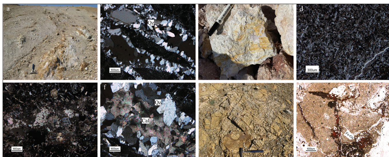
شکل ۱۰- دگرسانی‌های گرمایی در منطقه مورد مطالعه: (a) رگه ضخیم سیلیس، (b) تصویر میکروسکوپی از رگه سیلیسی (XPL)، (c) نمونه دستی مربوط به دگرسانی آرژیلیکی، (d) زمینه دگرسان شده در مقطع میکروسکوپی (XPL)، (e) دگرسانی کربناتی به صورت پراکنده در زمینه (XPL)، (f) رگه تاخیری کربناتی (XPL)، (g) برونزد اکسید آهن به صورت استوک‌ورکی، (h) اکسید آهن در مقاطع میکروسکوپی (PPL). Cal= کلسیت، Fe-Ox= اکسید آهن، QZ: کوارتز (Whitney and Evans, 2010).
