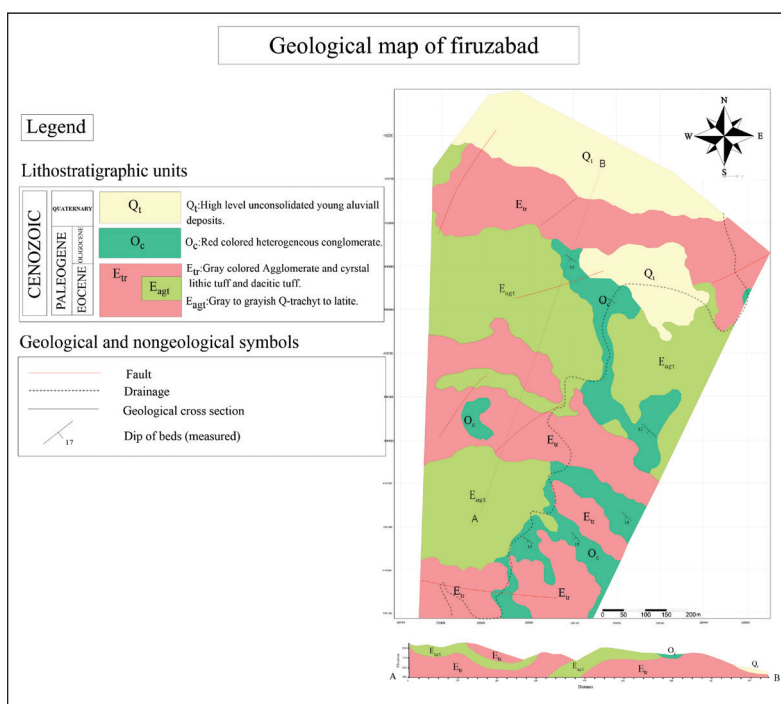
شکل ۱- نقشه زمین‌شناسی منطقه فیروزآباد (شرکت آذر ساروج سبلان، ۱۴۰۲).
