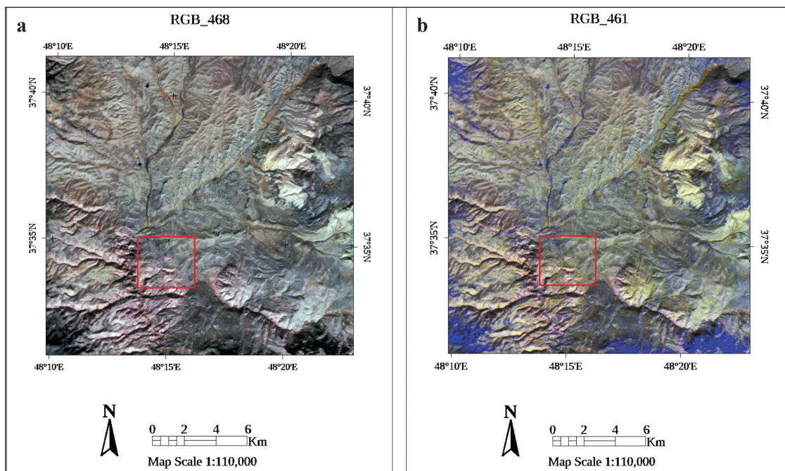
شکل ۲- تصاویر ترکیب رنگی کاذب سنجنده استر منطقه مورد مطالعه: (a) RGB-468 که مناطق صورتی رنگ در منطقه مورد مطالعه نشان دهنده دگرسانی آرژیلیک در منطقه می‌باشد. (b) RGB-461؛ در منطقه مورد مطالعه مناطق متمایل به صورتی نشانگر دگرسانی آرژیلیک و مناطق سبز روشن نشان دهنده اکسید آهن در منطقه می‌باشند. مناطق دارای رنگ آبی در حاشیه تصویر پوشش ابری بوده و مربوط به دگرسانی پروپلیتیک در منطقه نمی‌باشند.
