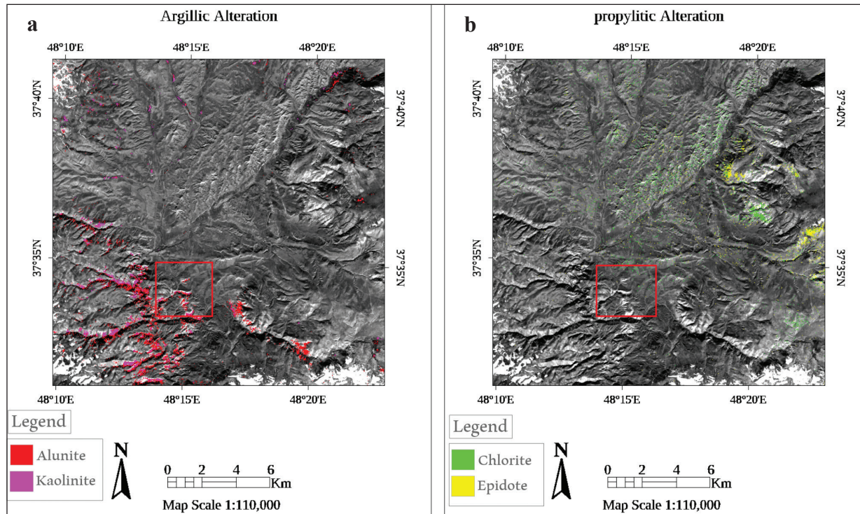
شکل ۸- پردازش تصاویر سنجنده استر به روش نقشه برداری زاویه طیفی: (a) بارزسازی کانی‌های شاخص پهنه دگرسانی آرژیلیک، (b) بارزسازی کانی‌های شاخص پهنه دگرسانی پروپلیتیک.
