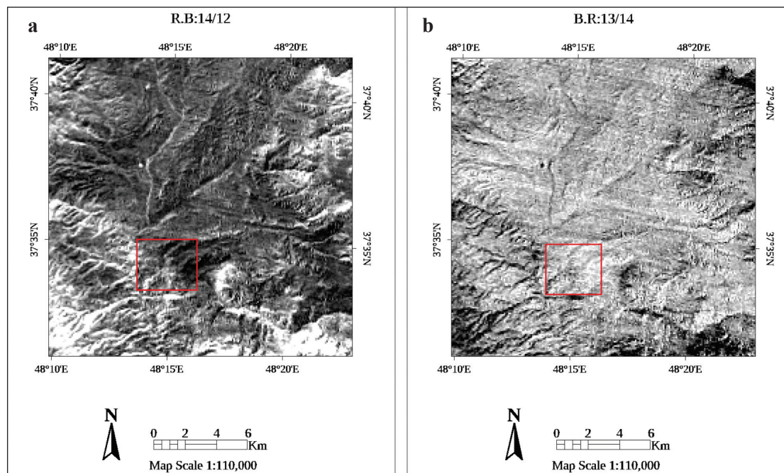
شکل ۵- پردازش تصاویر سنجنده استر: (a) نسبت گیری باندهای ۱۴ به ۱۲؛ پیکسل‌های روشن نشان‌دهنده مناطق دگرسانی سیلیسی می‌باشند. (b) نسبت گیری باندهای ۱۴ به ۱۳؛ پیکسل‌های روشن نشان‌دهنده دگرسانی کربناتی در منطقه می‌باشند.
