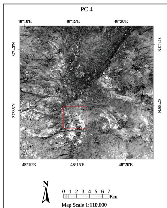
شکل ۷- پردازش تصاویر سنجنده لندست به روش کروستا؛ تصویر (PC4) مربوط به ترکیب باندهای ۲، ۴، ۵، ۶ پیکسل‌های روشن در تصویر نشان‌دهنده اکسید آهن در منطقه می‌باشند.
