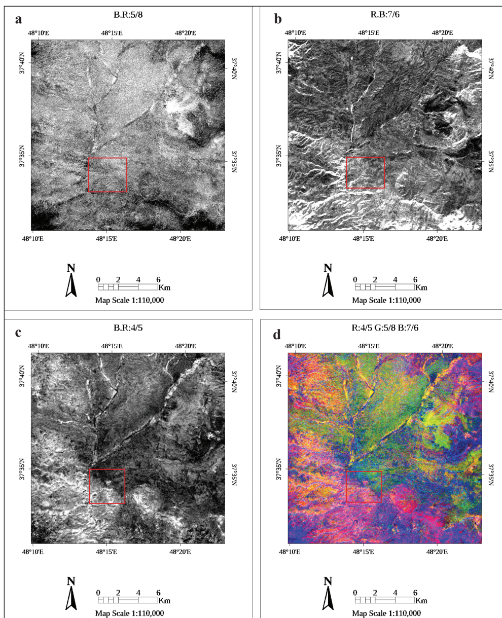
شکل ۴- پردازش تصاویر سنجنده استر: (a) روش نسبت گیری باند ۵ به ۸؛ پیکسل‌های روشن در تصویر نشان‌دهنده دگرسانی پروپلیتیک در منطقه می‌باشند. (b) نسبت گیری باندهای ۷ به ۶؛ پیکسل‌های روشن نشان‌دهنده دگرسانی فلیک در منطقه می‌باشند. (c) نسبت گیری باندهای ۴ به ۵؛ پیکسل‌های روشن نشان‌دهنده دگرسانی آرژیلیک در منطقه می‌باشند. (d) ترکیب رنگی R:4/5 G:5/8 B:7/6 که در منطقه مورد مطالعه مناطق قرمز تا صورتی رنگ نشانگر دگرسانی آرژیلیکی می‌باشند.
