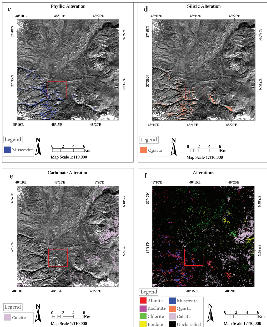
ادامه شکل ۸- پردازش تصاویر سنجنده استر به روش نقشه‌برداری زاویه‌طیفی: (c) بارزسازی کانی‌های شاخص پهنه دگرسانی فلیک، (d) بارزسازی کانی‌های شاخص پهنه دگرسانی سیلیسی، (e) بارزسازی کانی‌های شاخص دگرسانی کربناتی، (f) بارزسازی دگرسانی‌های موجود در منطقه مورد مطالعه؛ کانی‌های شاخص هر پهنه با رنگ‌های متفاوت نمایش داده شده‌اند.
