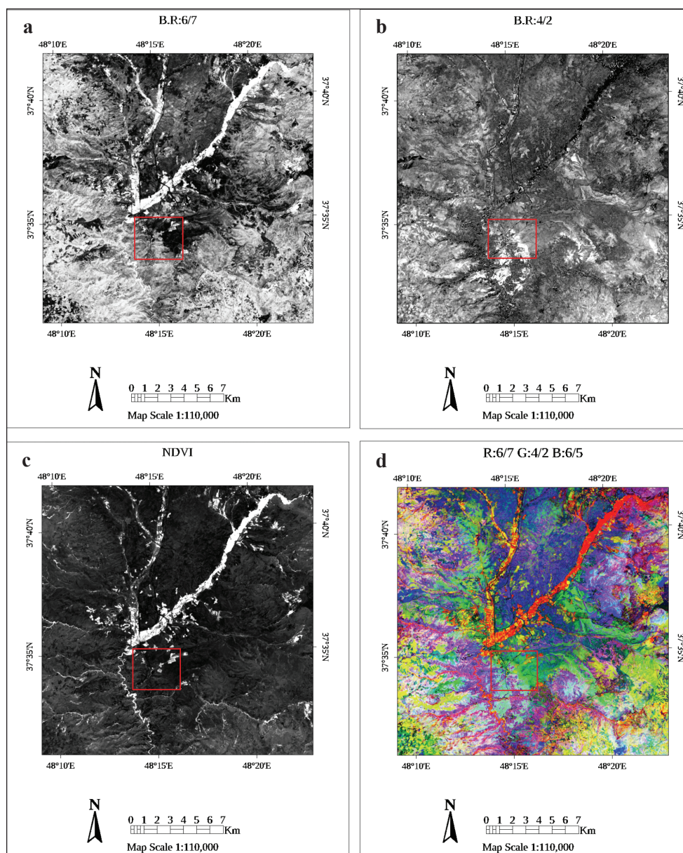
شکل ۳- پردازش تصاویر سنجنده لندست: (a) روش نسبت گیری باند ۶ به ۷؛ پیکسل‌های روشن در تصویر نشان‌دهنده مناطق دگرسانی در منطقه می‌باشند. (b) نسبت گیری باندهای ۴ به ۲؛ پیکسل‌های روشن نشان‌دهنده مناطق اکسید آهن می‌باشند. (c) شاخص NDVI که در تصویر حاصل، پیکسل‌های روشن نشان‌دهنده پوشش گیاهی در منطقه می‌باشند. (d) ترکیب رنگی R:6/7 G:4/2 B:6/5 که در منطقه مورد مطالعه، مناطق صورتی رنگ نشانگر دگرسانی آرژیلیکی می‌باشند.
