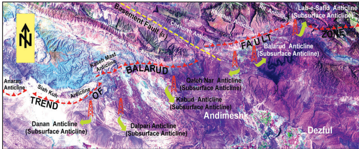
شکل ۶- تصویر ماهواره‌ای محدوده شمال اندیمشک و دزفول برای نمایش آرایش پوششی قطعات بسیار منطقه گسلی بالارود. در این تصویر موقعیت تاقدیس‌های روسطحی و زیرسطحی متأثر از عملکرد منطقه گسلی بالارود مشخص شده است. \alpha موقعیت گسل پی‌سنگی معرفی شده در شکل ۴ را نشان می‌دهد. به جابه‌جایی روند گسل بالارود توسط این گسل توجه شود. موقعیت این تصویر در شکل ۱ مشخص شده است.
