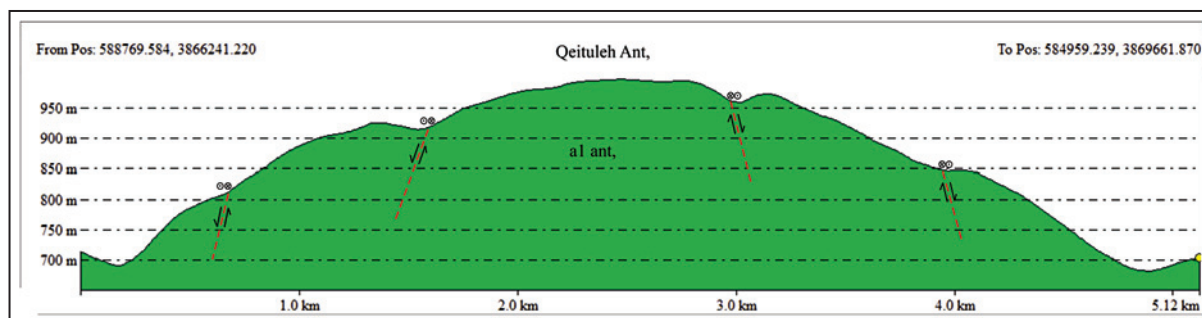
شکل ۷- هندسه پله ای و گسترش گسلش عادی در مقطع طولی از چین a1 تا قدیس قیتوله.
