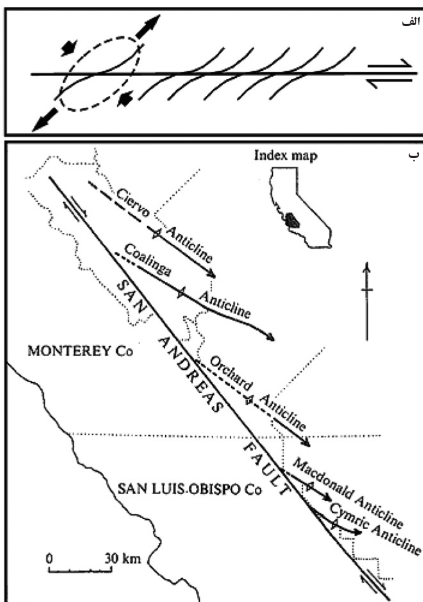
شکل ۵- الف) نمودار نمادین که پیش‌بینی راستای محور چین‌های تشکیل شده در بالای گسل پی‌سنگی راست گرد را نشان می‌دهد (منحنی خطوط مایل)؛ ب) چین‌های پلکانی بالای گسل سان‌آندریاس (برگرفته از (Price & Cosgrove (1990)).
