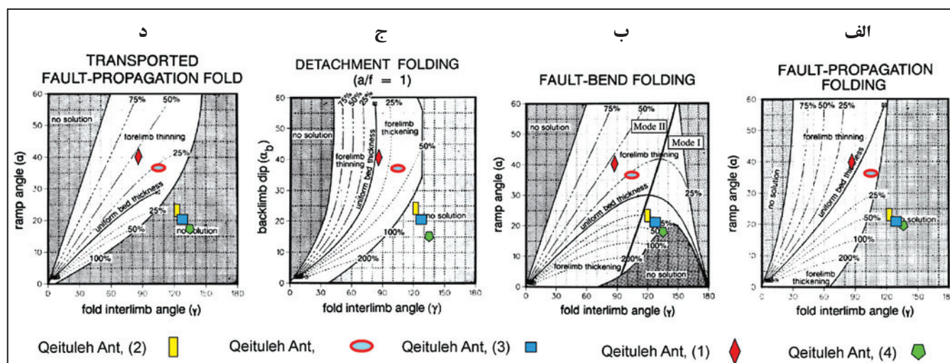
شکل ۳- نمودار سترشدگی و نازک‌شدگی پهلوی پیشانی برای چین‌های: الف) گسترش گسلی حمل‌شده؛ ب) خمش گسلی؛ ج) جدایشی؛ د) گسترش گسلی (انتشاری) و موقعیت چین‌های تاق‌دیس قیتوله در این نمودارها (برگرفته از (Jamison 1987).
