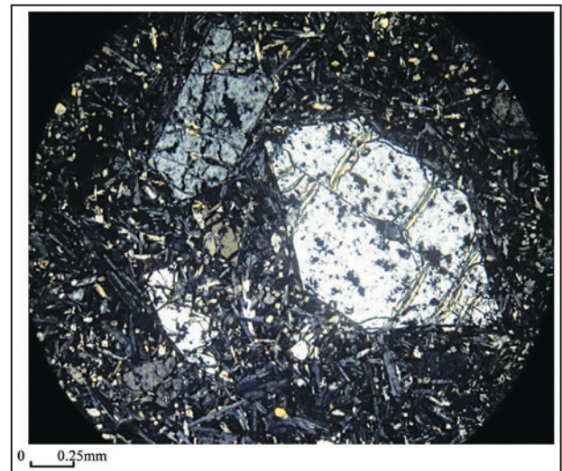
شکل ۳- نمایی از بافت پورفیریک با خمیره میکروولیتی در گدازه بالشی با ترکیب اولوین بازالت. همان‌طور که مشخص است فنوکریست‌های اولوین سالم بوده و تنها در امتداد شکستگی‌های خود تبدیل به سرپانتین شده‌اند.
