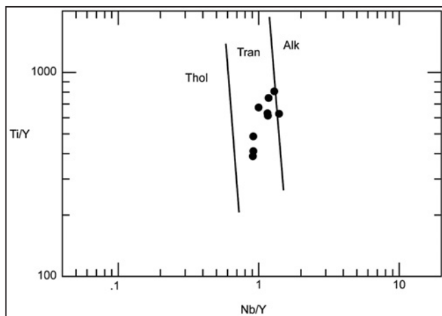
شکل ۶- موقعیت بازالت‌های بالشی منطقه در تقسیم‌بندی (Pearce 1982).
