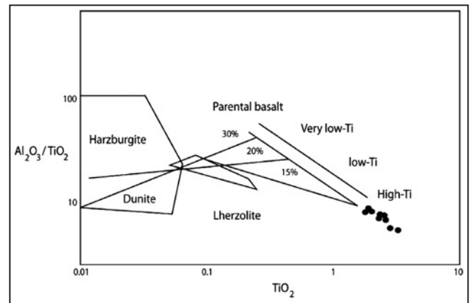
شکل ۱۹ - موقعیت بازالت‌های بالشی در نمودار لگاریتمی Al_2O_3/TiO_2 در برابر TiO_2 از Beccaluva et al. (1983).
