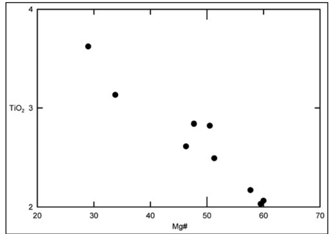
شکل ۹- موقعیت بازالت‌های بالشی منطقه در نمودار TiO_2 در برابر Mg\# .
