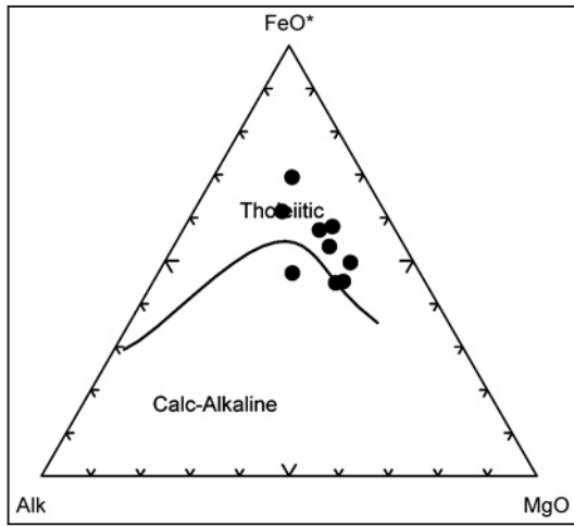
شکل ۱۰- موقعیت بازالت‌های بالشی منطقه در نمودار AFM.
