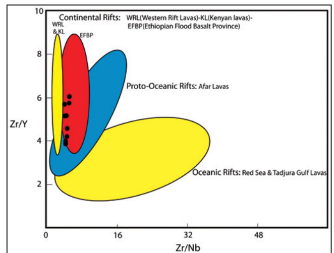
شکل ۲۱ - موقعیت بازالت‌های بالشی در نمودار Zr/Y در برابر Zr/Nb (Kampunzu & Mohr, 1991).
