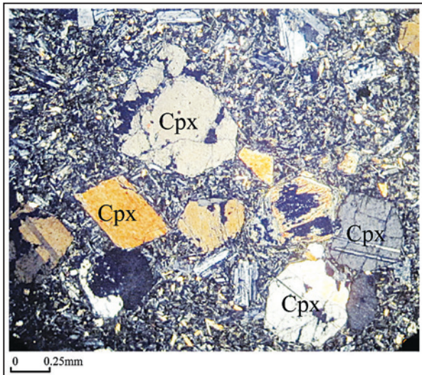
شکل ۴- بافت پورفیریک با خمیره میکروولیتی در گدازه بالشی با ترکیب بازالت. فراوانی فنوکریست‌های کلینوپروکسن (Cpx) و فقدان اولوین از ویژگی‌های این پیلوها است.
