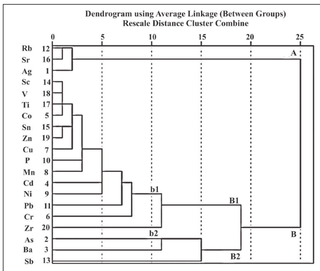
شکل ۶- نمودار تحلیل خوشه‌ای عناصر مورد مطالعه در رسوبات سطحی ناحیه خور و بیابانک.
