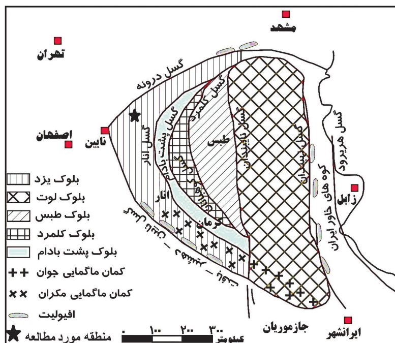
شکل ۲- خردقاره ایران مرکزی و زیر پهنه‌ی آن (آقائاتی، ۱۳۸۹).
