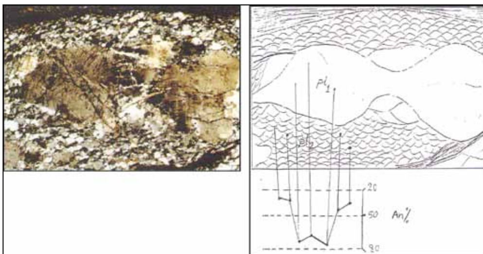
شکل ۱۵- تغییرات مؤلفه آنورتیتی پلاژیو کلازا ضمن فرایند میلوئیتی شدن، بزرگنمایی ۴۰، (Pl 1 = پلاژیو کلاز اولیه، Pl 2 = پلاژیو کلاز نوزاد)
