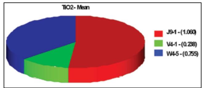
شکل ۹ - مقایسه TiO 2 آمفیبول‌های اولیه (V 4 -1)، آمفیبول‌های حاصل از دگرشکلی (J 9 -1) و آمفیبول‌های حاصل از متاسوماتیسم (W 4 -5)
