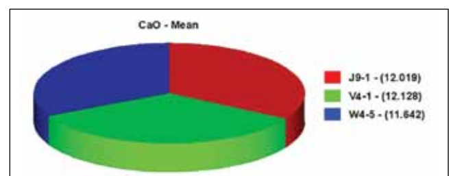
شکل ۷- مقایسه CaO آمفیبول‌های اولیه (V 4 -1)، آمفیبول‌های حاصل از دگرشکلی (J 9 -1) و آمفیبول‌های حاصل از متاسوماتیسم (W 4 -5)
