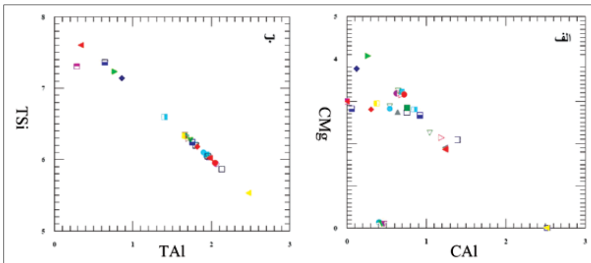
شکل ۱۲ - نمایش واکنش چرماکتی ( Al^{VI}Al^{IV} = Mg^{VI}Si^{IV} )، الف) با افزایش Al در موقعیت تراهدر از میزان Si کاسته می‌شود. ب) با افزایش Al در موقعیت اکتاهدر از میزان Mg در این جایگاه کاسته می‌شود (نشانه نمونه‌ها مشابه شکل ۱۱ هستند).
