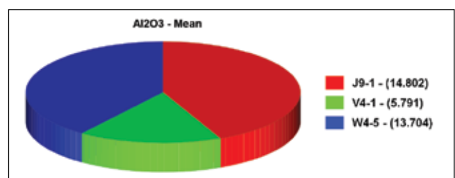
شکل ۵- مقایسه Al 2 O 3 آمفیبول‌های اولیه (V 4 -1)، آمفیبول‌های حاصل از دگرشکلی (J 9 -1) و آمفیبول‌های حاصل از متاسوماتیسم (W 4 -5)
