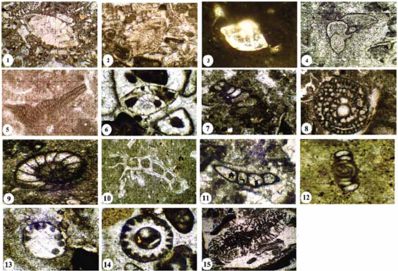
Fig. 1&2: Miscellanea miscella , Sample.No:P.R:16,24. Fig. 3: Rotalia ( aff Rotalia provalis ), Sample.No:P.R:5. Fig. 4: Cibicides gr lobatus , Sample.No:P.R:8. Fig. 5: Distichoplax biserialis , Sample.No:P.R:35. Fig. 6: Kathina sp., Sample.No:P.R:41. Fig. 7: Textularides sp., Sample.No:P.R:38. Fig. 8: Alveolina (Glomalveolina) . Sample.No:P.R:51.
