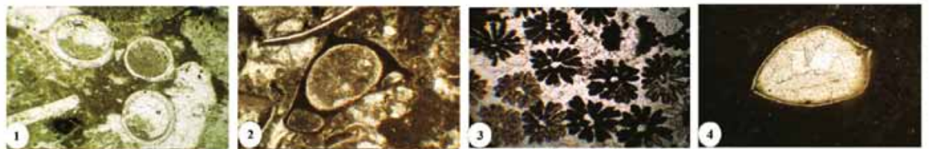
Fig 1: Serpula sp. Sample.No:P.R:111. Fig 2: worm tube , Sample.No:P.R:142.
