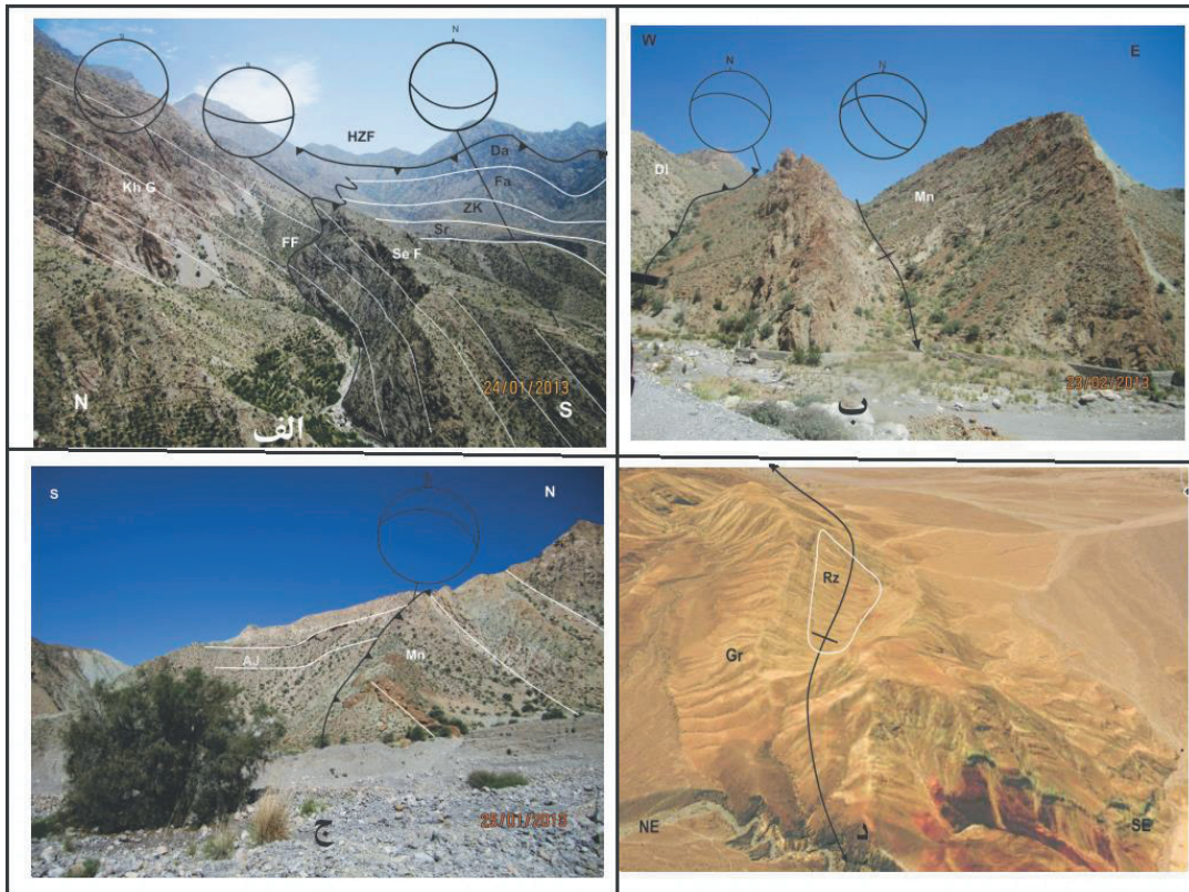
شکل ۹- ساختارهای دیده شده در تاقدیس فراقان (عکس‌ها در دره زکین گرفته شده است که به صورت مستطیل آبی در شکل ۲ دیده می‌شود): الف) رانده شدن سازند سیاهو (Se F) در امتداد گسل فراقان (به عنوان ینگ گسل پس‌راند با سوی شیب شمال‌خاوری) روی گروه خامی (KhG) در فاز دگرشکلی ۱. در این شکل سازندهای فراقان، زکین، سرچاهان و دالان به ترتیب با نمادهای Zk، Fa، Da نمایش داده شده‌اند؛ ب) رانده شدن سازند میشان (Mn) روی سازند دالان (DI) در امتداد HZF و چین‌های جدایشی حاصل از فعالیت پهنه جدایش میانی پابده و گوری در فرودپواره گسل در فاز ۲؛ ج) رانده شدن سازند میشان (Mn) روی سازند آغاچاری در امتداد یک رانده‌گی میان بر فرودپواره‌ای در فاز ۲؛ د) نمایی از تاقدیس کوچک فرودپواره آبی ناشی از فعالیت زون جدایش میانی پابده و گوری در فرودپواره گسل HZF در فاز ۲. سازندهای رازک و بخش گوری سازند میشان به ترتیب با نمادهای Gr و Rz نمایش داده شده‌اند.
