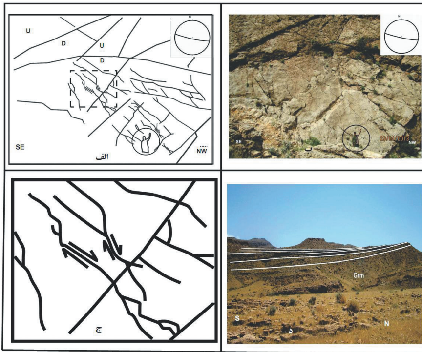
شکل ۷- الف و ب) فعالیت دوباره شکستگی‌ها در نزدیکی ایستگاه S1 در سازند جهرم؛ ج) فعال شدن شکستگی‌های اولیه به صورت گسل‌های راست‌گرد کوچک؛ د) چینه‌های رشدی در پیرامون گنبد نمکی دماغه خاوری ناقدیس فراقان.
