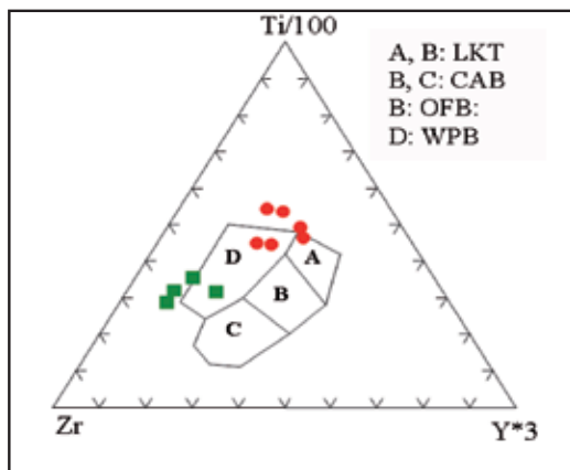
شکل ۸- نمودار متمایز کننده Ti-Zr-Y برای بازالت‌ها (Pearce & Cann, 1973). LKT: تولیت‌هایی با پتاسیم کم، CAB: بازالت‌های کلسیمی-قلیایی، OFB: بازالت‌های کف اقیانوسی و WPB: بازالت‌های درون‌صفحه‌ای، [اعلامیم مانند شکل ۵ است].
