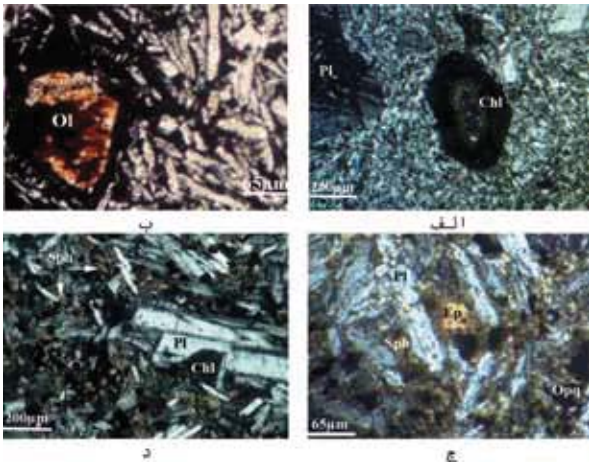
شکل ۴- تصاویر میکروسکوپی مربوط به سنگ‌های آتشفشانی سیلورین در تاق‌دیس جهت (بجز تصویر الف که در نور PPL گرفته شده است، بقیه تصاویر مربوط به نور XPL هستند). الف و ب) کانی‌های فرومیزین که توسط کانی‌های ثانویه‌ای همچون کلریت جانشین شده‌اند، ج و د) همراهی فلدسپات با کلریت، اپیدوت، اسفن و اپاک را نشان می‌دهد.
