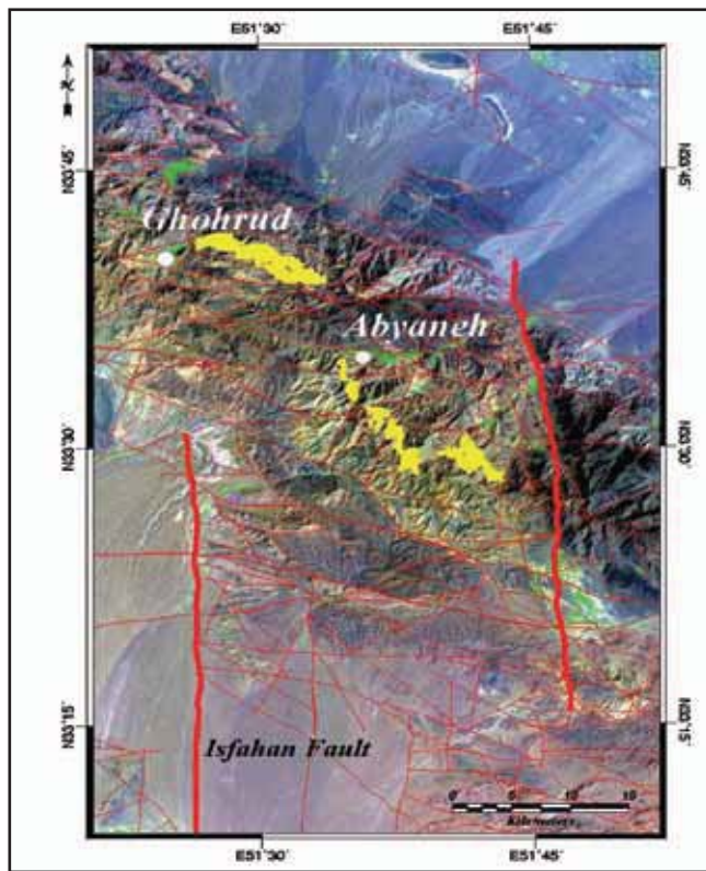
شکل ۱۰- تصویر حاصل از پردازش داده‌های رقومی TM به صورت RGB=741 پس از ایجاد کشیدگی خطی ۹۹٪ بر روی هر باند. گسل‌های شناسایی شده در منطقه، با خطوط سرخ‌رنگ و رخنمون سنگ‌های آتشفشانی سیلورین، با رنگ زرد مشخص شده‌اند.
