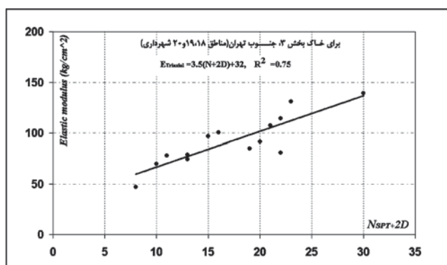
شکل ۵- رابطه میان E و N برای بخش ۳، بر مبنای نتایج آزمون سه محوری
