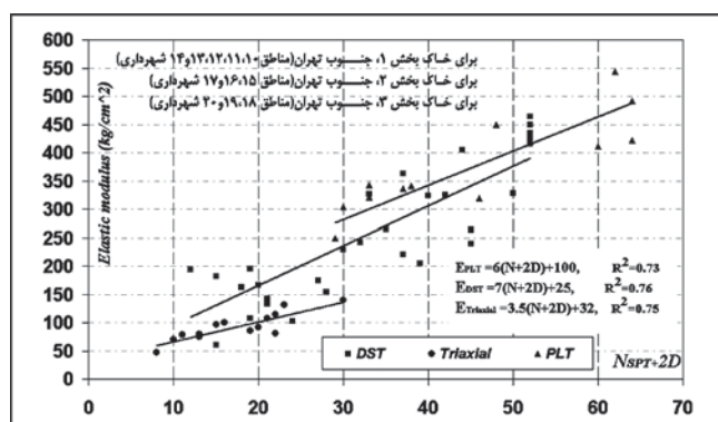
شکل ۶- رابطه میان E و N برای هر سه بخش مورد مطالع در جنوب تهران
