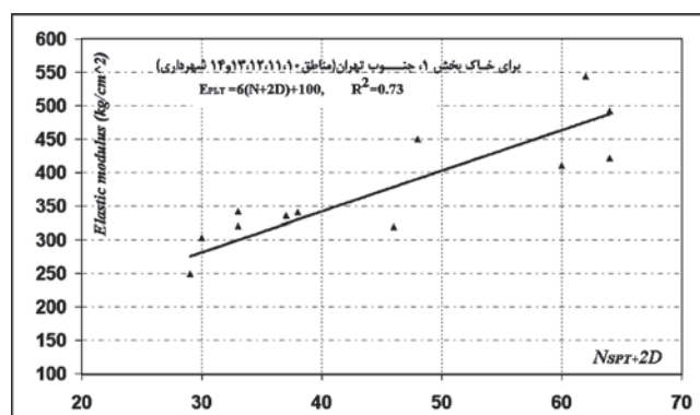
شکل ۳- رابطه میان E و N برای بخش ۱، بر مبنای نتایج آزمون بارگذاری صفحه‌ای
