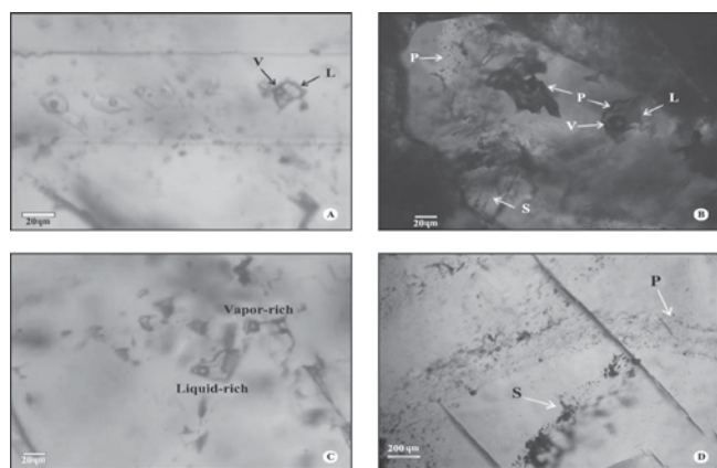
شکل ۶- (A) میانبارهای سیال اولیه در یک زون رشدی در کلسیت با نسبت‌های متفاوت بخار به مایع. (B) دو میانبار اولیه بزرگ در کوارتز که به صورت جدا از هم قرار گرفته‌اند. دیگر میانبارهای سیال در زون‌های رشدی (P) و در شکستگی‌های بسته شده (S) دیده می‌شود. (C) همزیستی فاز غنی از مایع و غنی از بخار در میانبارهای سیال اولیه نمونه کلسیتی ZK002-8. (D) میانبارهای اولیه در زون رشدی کلسیت که به وسیله شکستگی بسته شده حاوی میانبارهای ثانویه قطع می‌شود. اولیه: P؛ ثانویه: S؛ مایع: L؛ بخار: V
