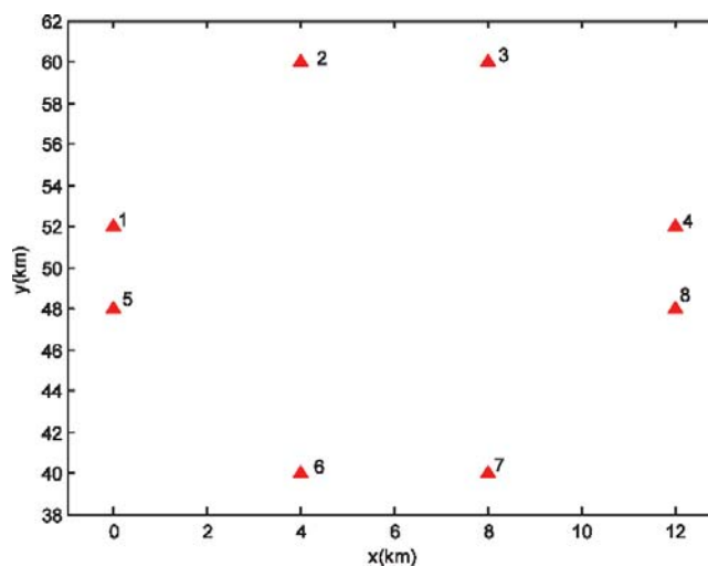
شکل ۳- شبکه اولیه با ۸ ایستگاه که در دو طرف گسل، در فاصله‌های \pm 10 ، \pm 2 کیلومتری قرار دارند
